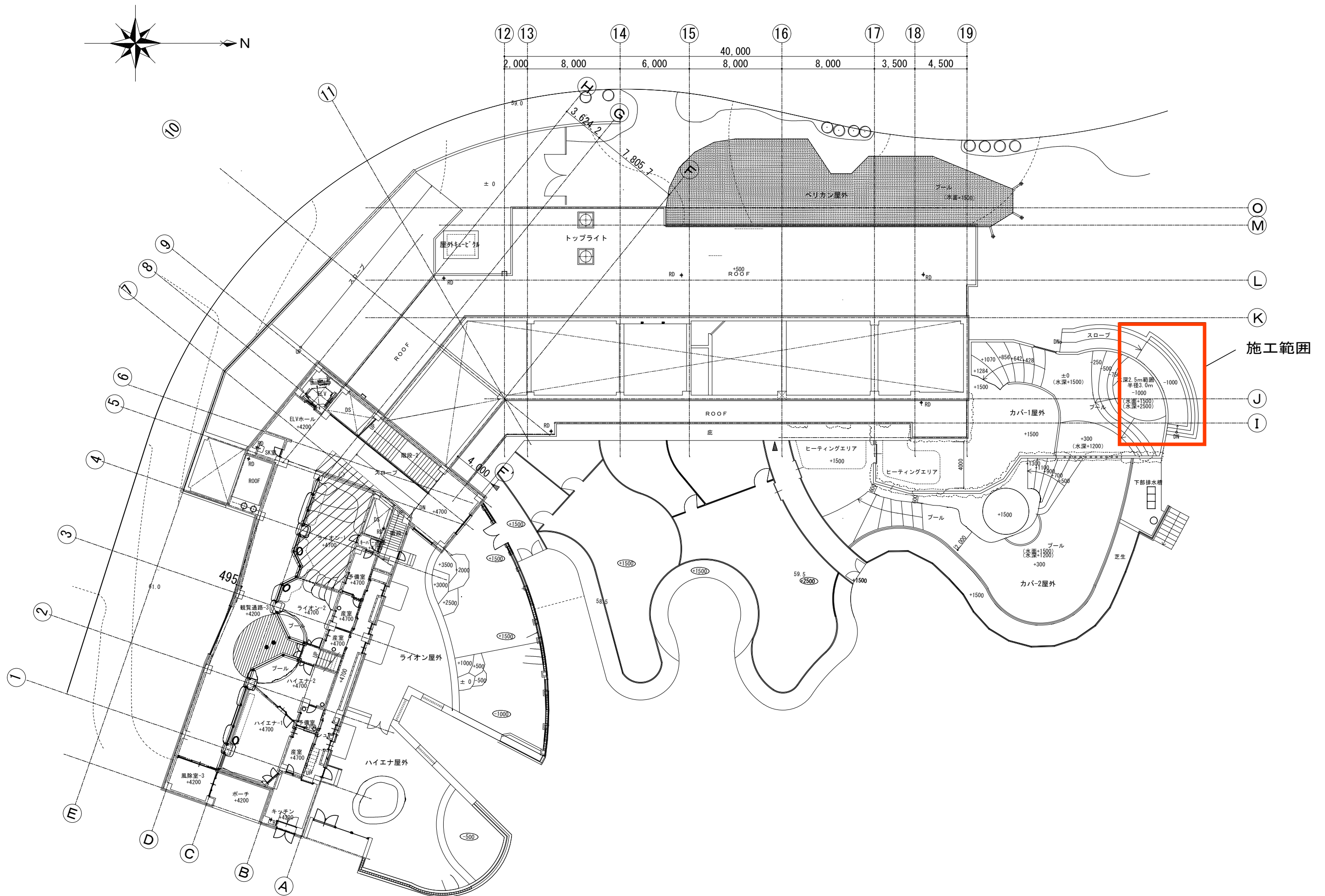
カバ・ライオン館2階及び屋外平面図
