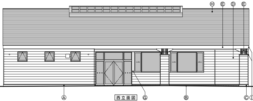
西立面図
