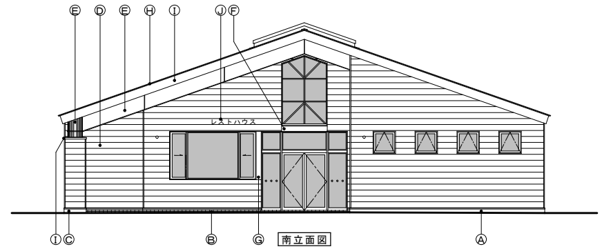
南立面図
