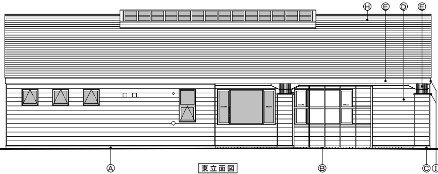
東立面図
