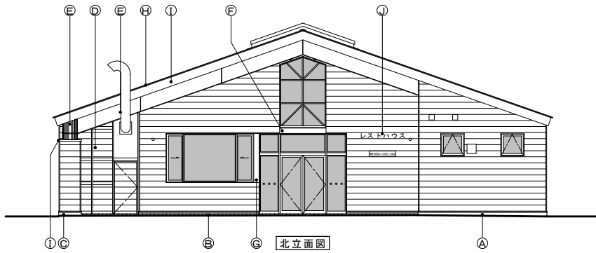
北立面図
