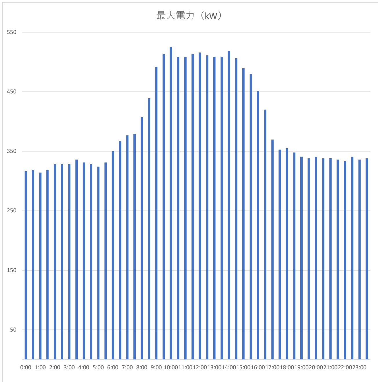
【最大需要電力発生日の負荷曲線図】 2024年3月2日
