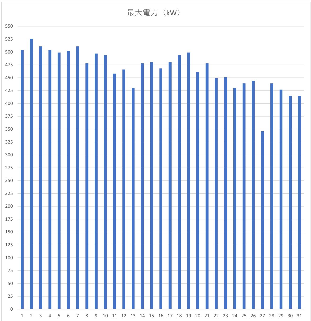
【最大需要電力発生月の負荷曲線図】2024年3月（2日最大需要電力発生日）
