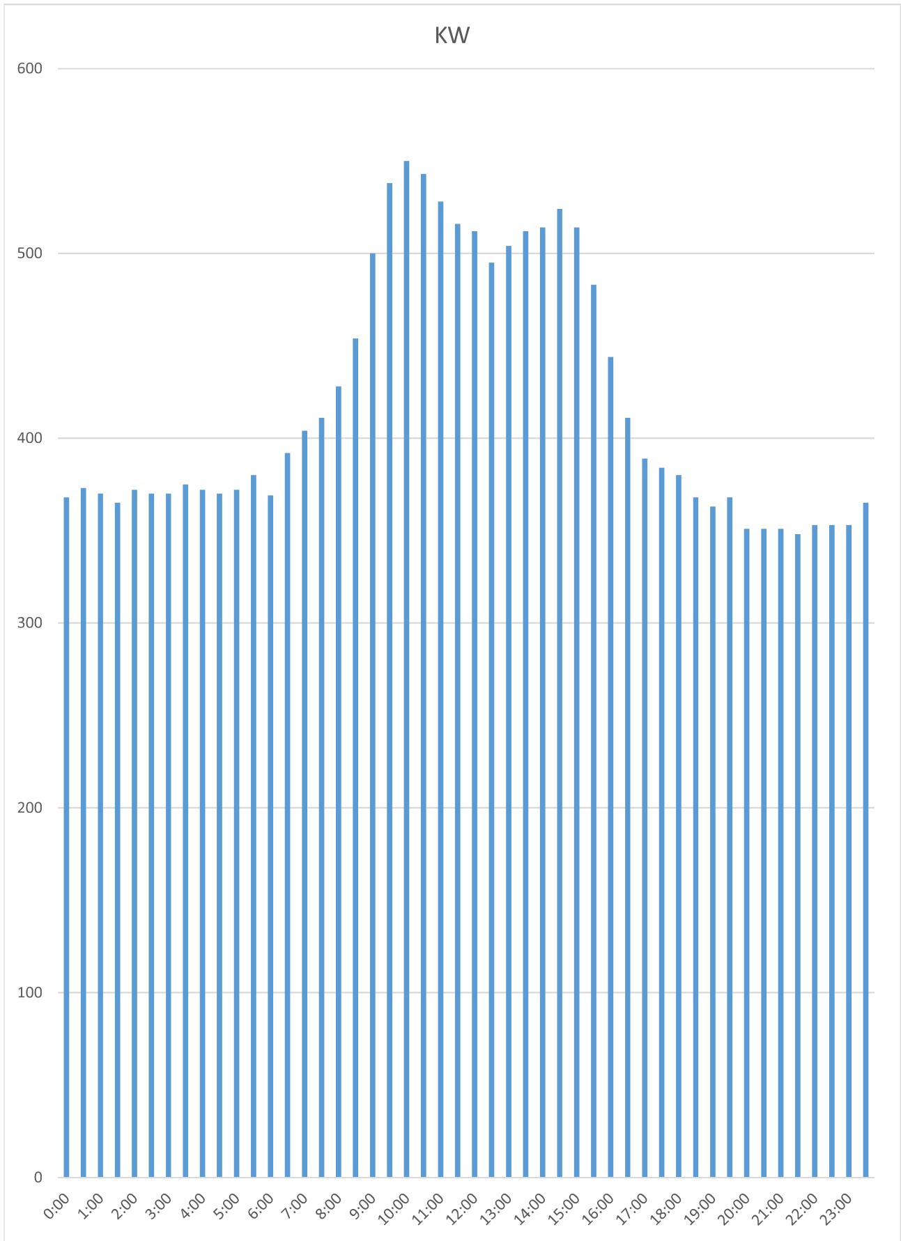
【最大需要電力発生日の負荷曲線図】 2023年1月26日
