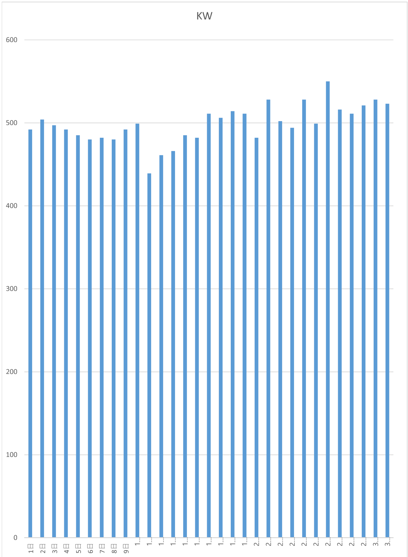
【最大需要電力発生月の負荷曲線図】 2023年1月（26日最大需要電力発生日）
