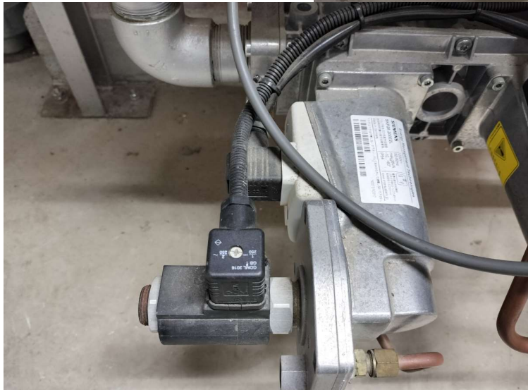
SKP26.200E2L 200V
