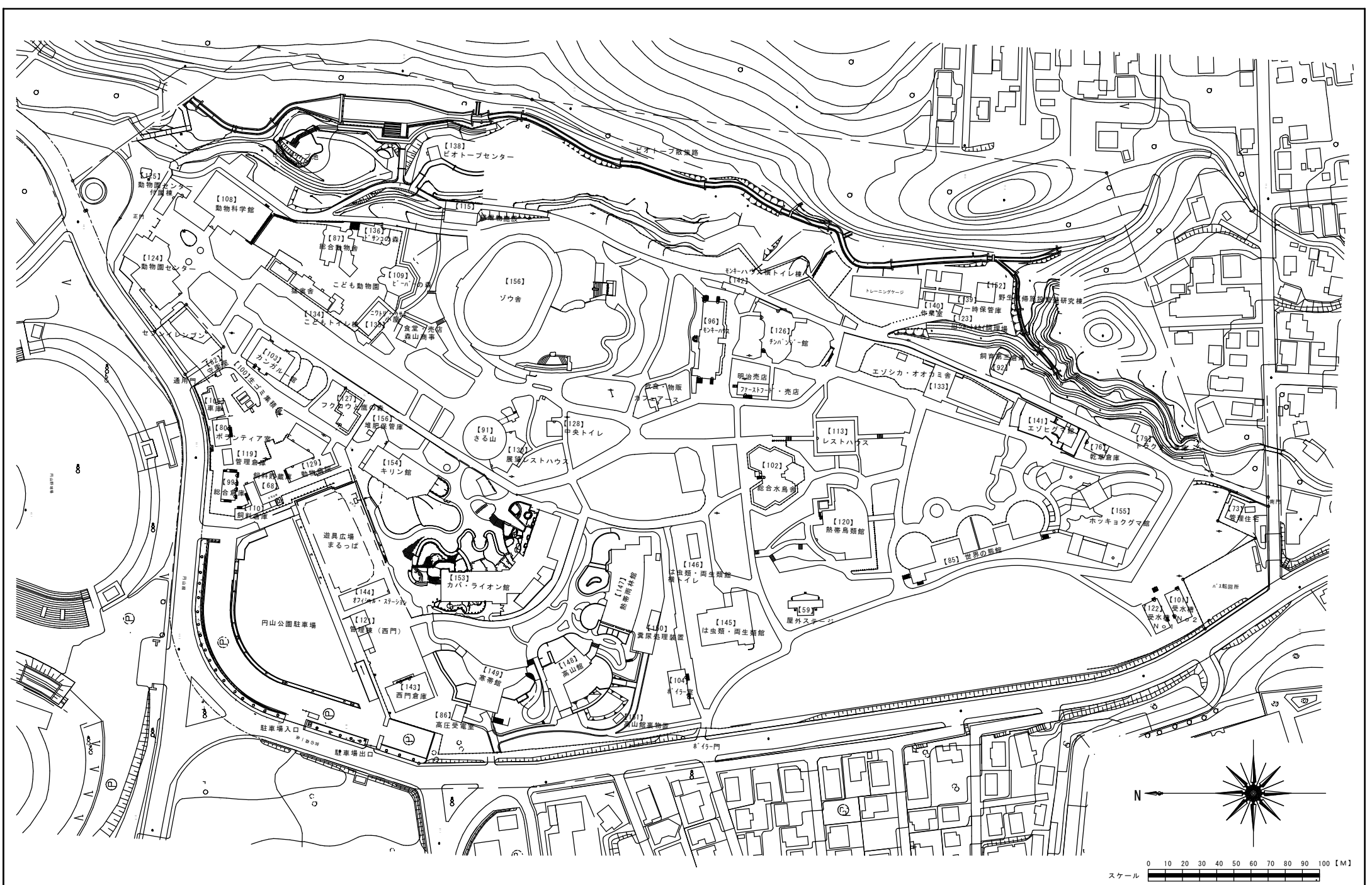
配置図 S=1/1,000
