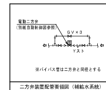
二方弁装置配管要領図 (補助水系統)
