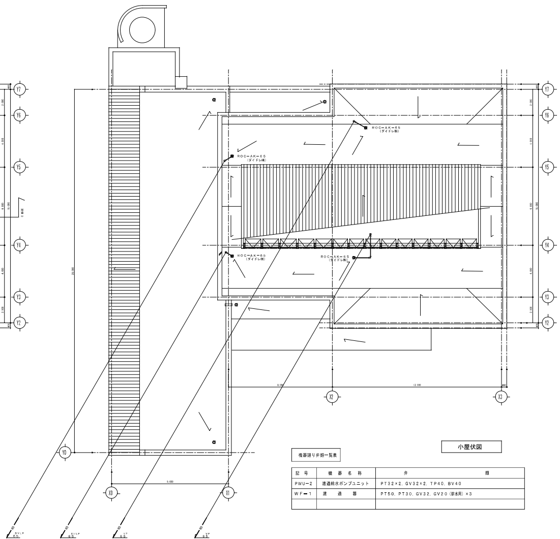
1-1階平面図
