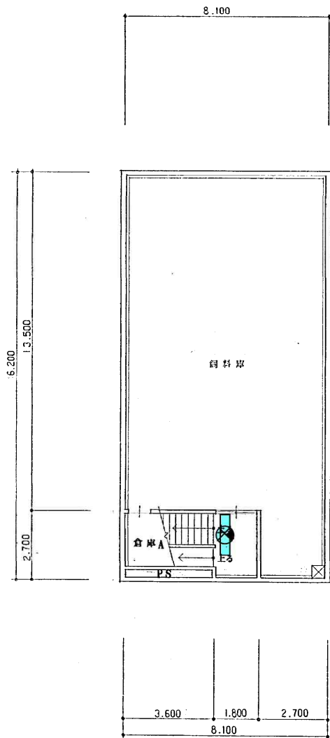
B1 階平面図
