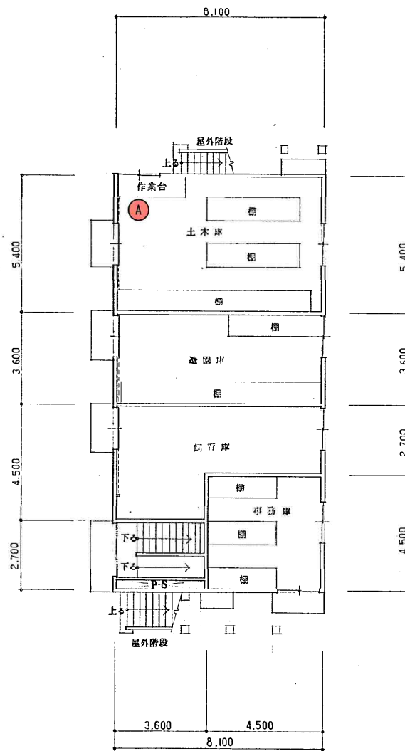
1 階平面図
