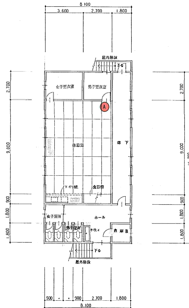
2 階平面図
