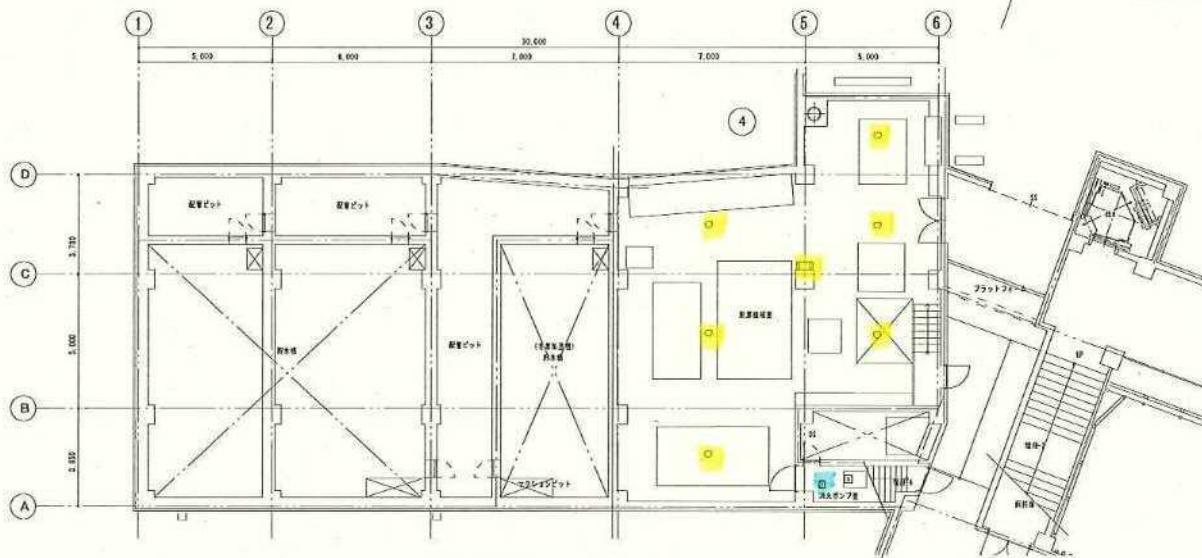
1階平面図-2 S=1/100
