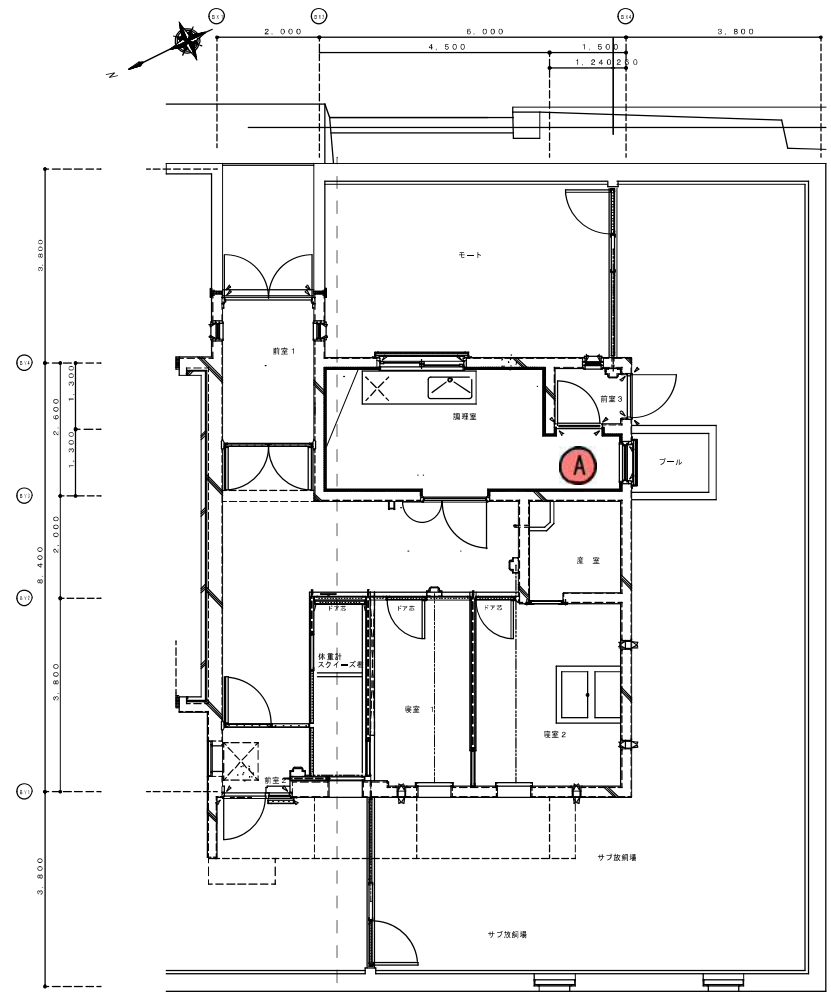
管理棟室平面詳細図 S=1/50
