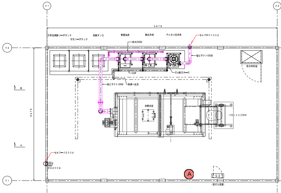
廃水処理設備 配管平面図 S=1/30
