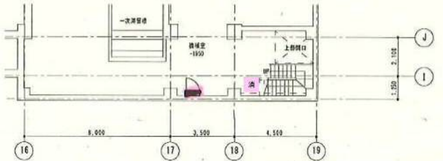
地階平面図 (衛生設備) S=1/100
