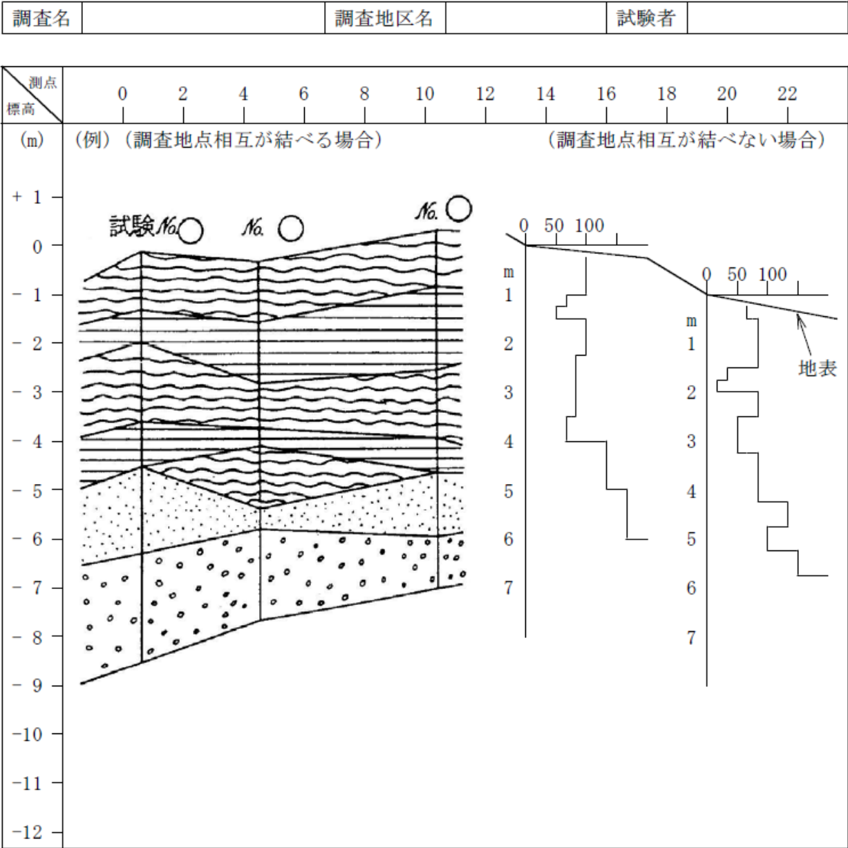
スクリーウエイト（スウェーデン式サウンディング）の貫入抵抗断面図
