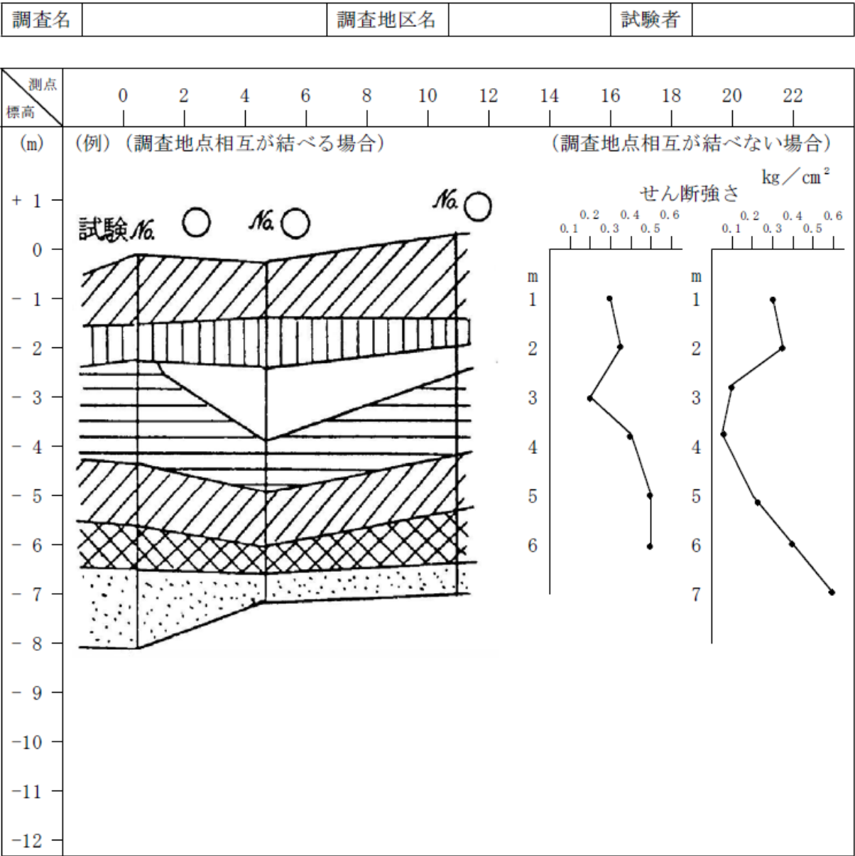
ベーンテストせん断強度断面図
