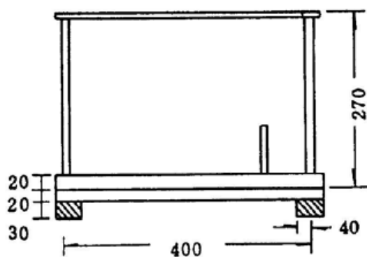
正面図
