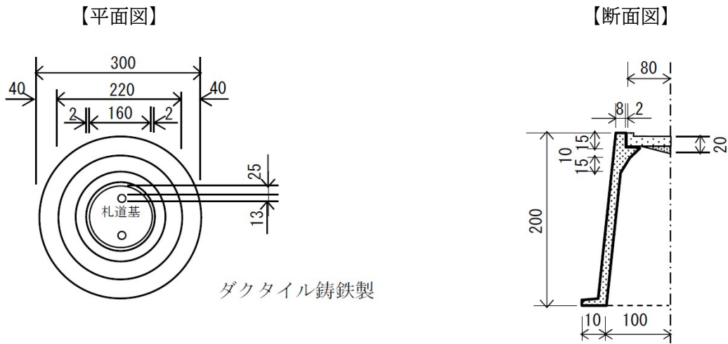
舗装路面用蓋 詳細図
