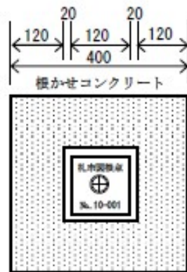
【ブロック類 詳細図】
