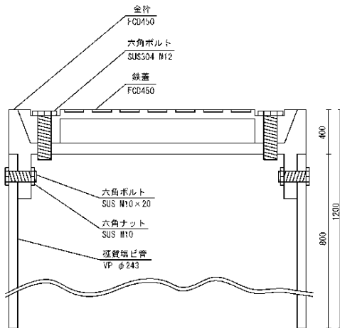
【公共基準点用鉄蓋（金棒・塩ビ管共）断面図】
