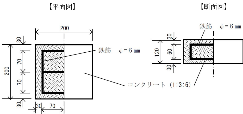
砂利道用蓋 詳細図
