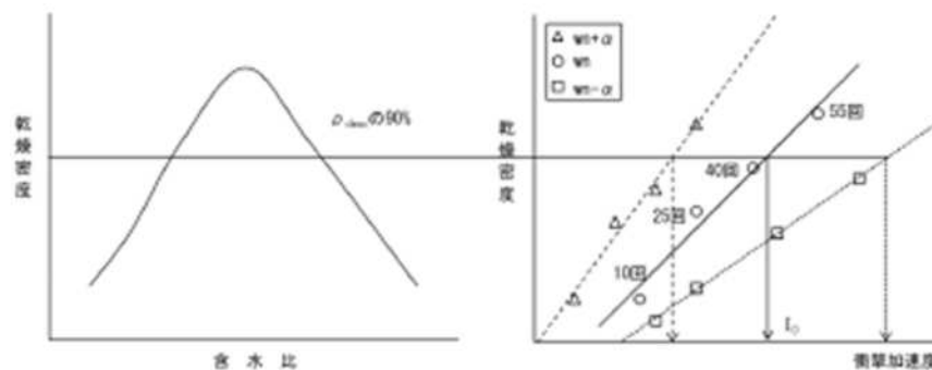
図 - 2.b 基準となる衝撃加速度（含水比が変わるおそれがある場合）
