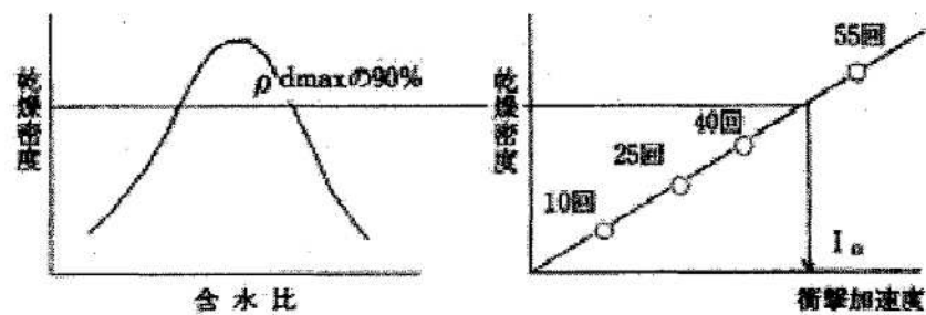
図 - 2.a 基準となる衝撃加速度
