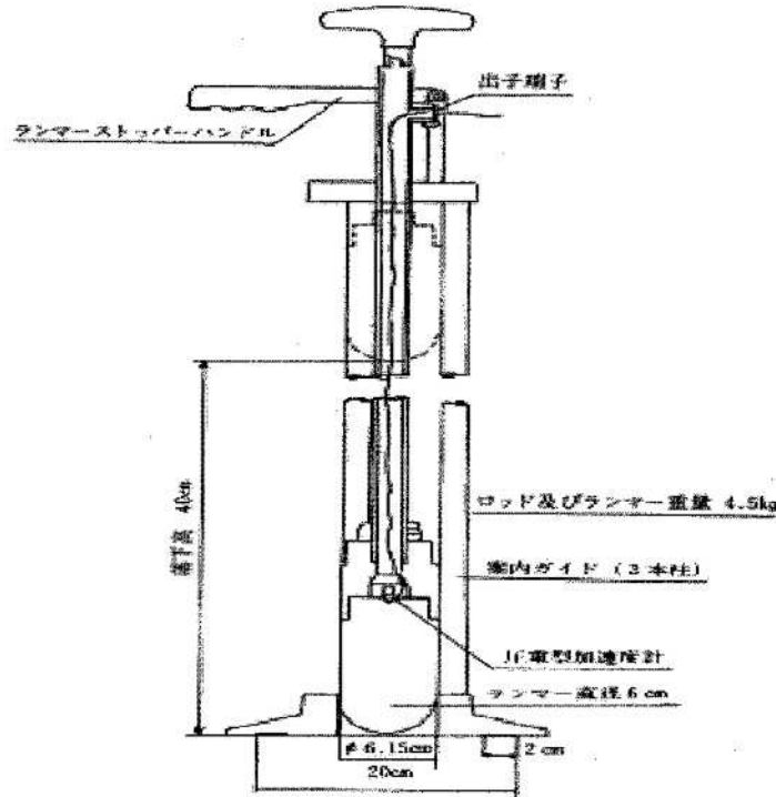
図 - 1 衝撃加速度測定装置
