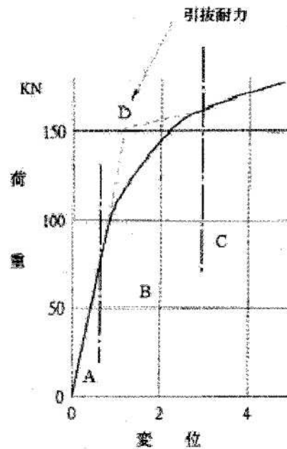
図1 ロックボルトの引抜試験
