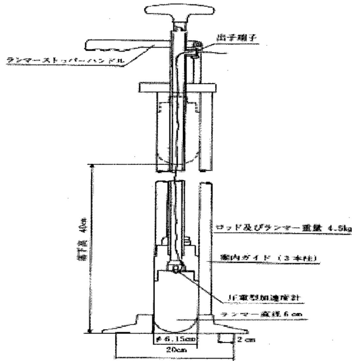
図－1 衝撃加速度試験器
