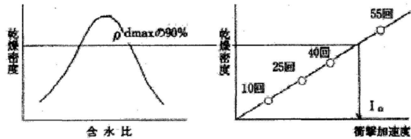
図－３ 締固め試験によって明確な最大乾燥密度が得られる試料の基準となる衝撃加速度
