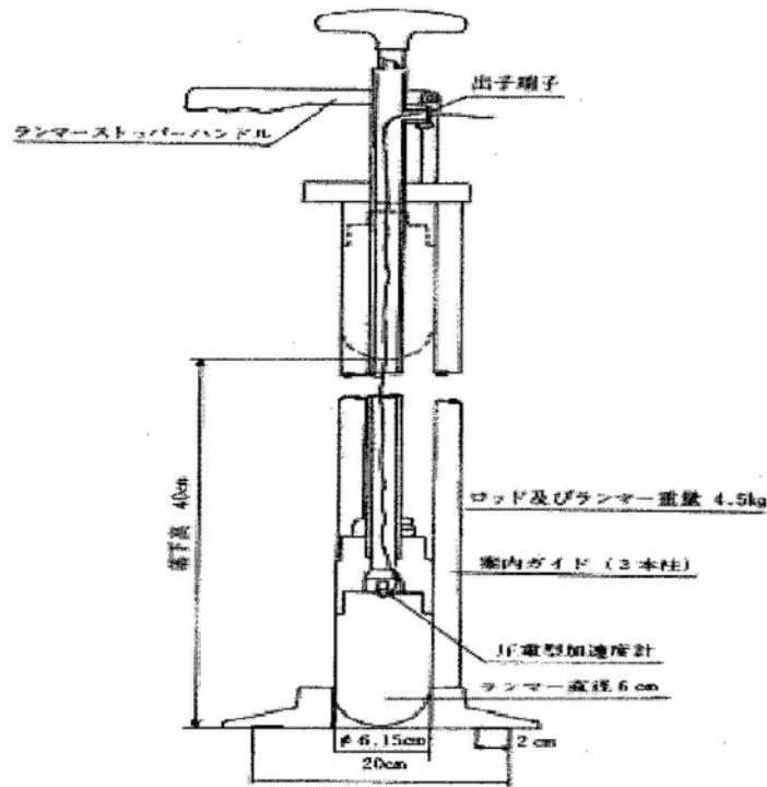
図－１ 衝撃加速度試験器
