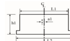
中心線の変位 (a1: 橋軸直角方向) (a2: 橋軸方向)
