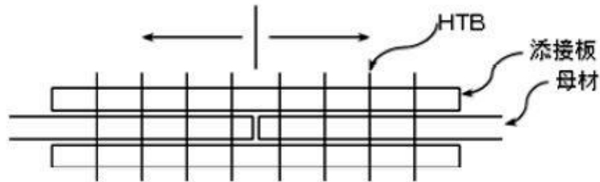
図 4 - 1 ボルト締め付け順序
