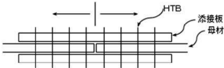
図 4-1 ボルト締め付け順序
