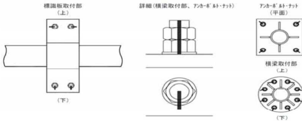
図3-2 合いマーク施工概念図
