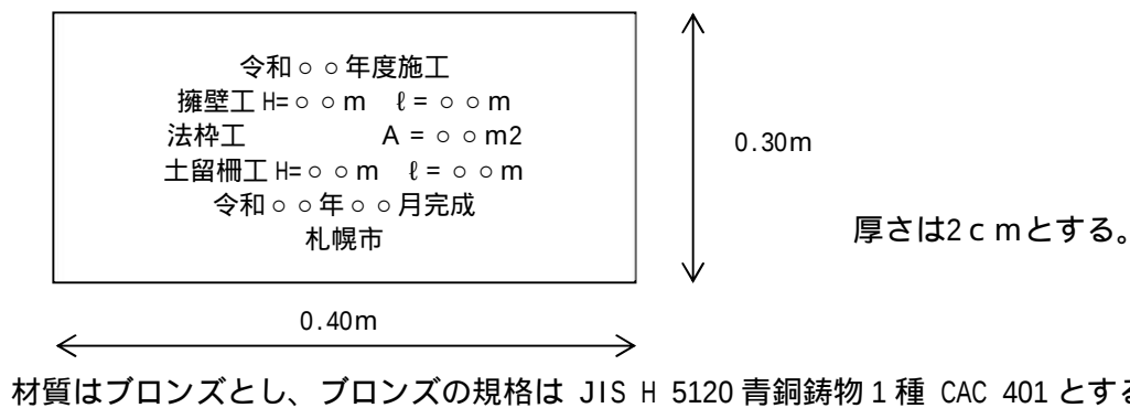
図 16 - 4 急傾斜用概要板
