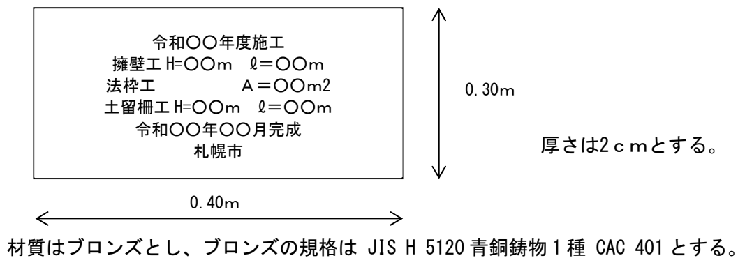
図 16-4 急傾斜用概要板
