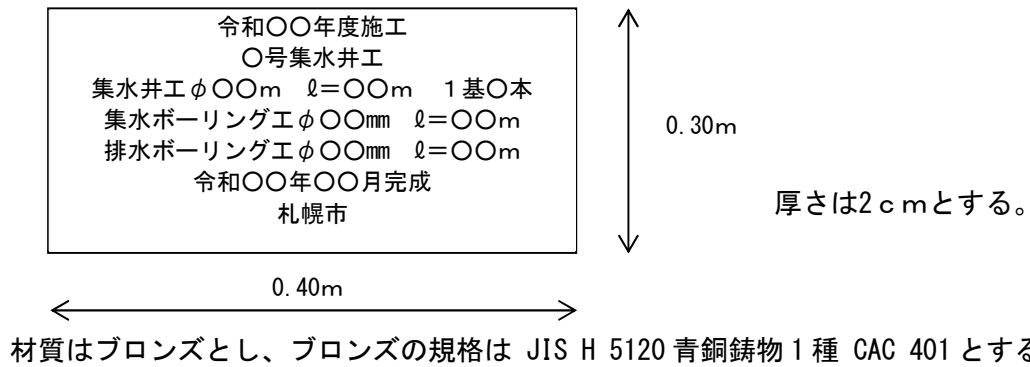
図 16-3 地すべり用概要板
