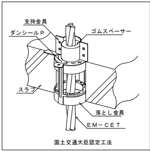
防火区画貫通処理 参考図 (※B(P S内))
