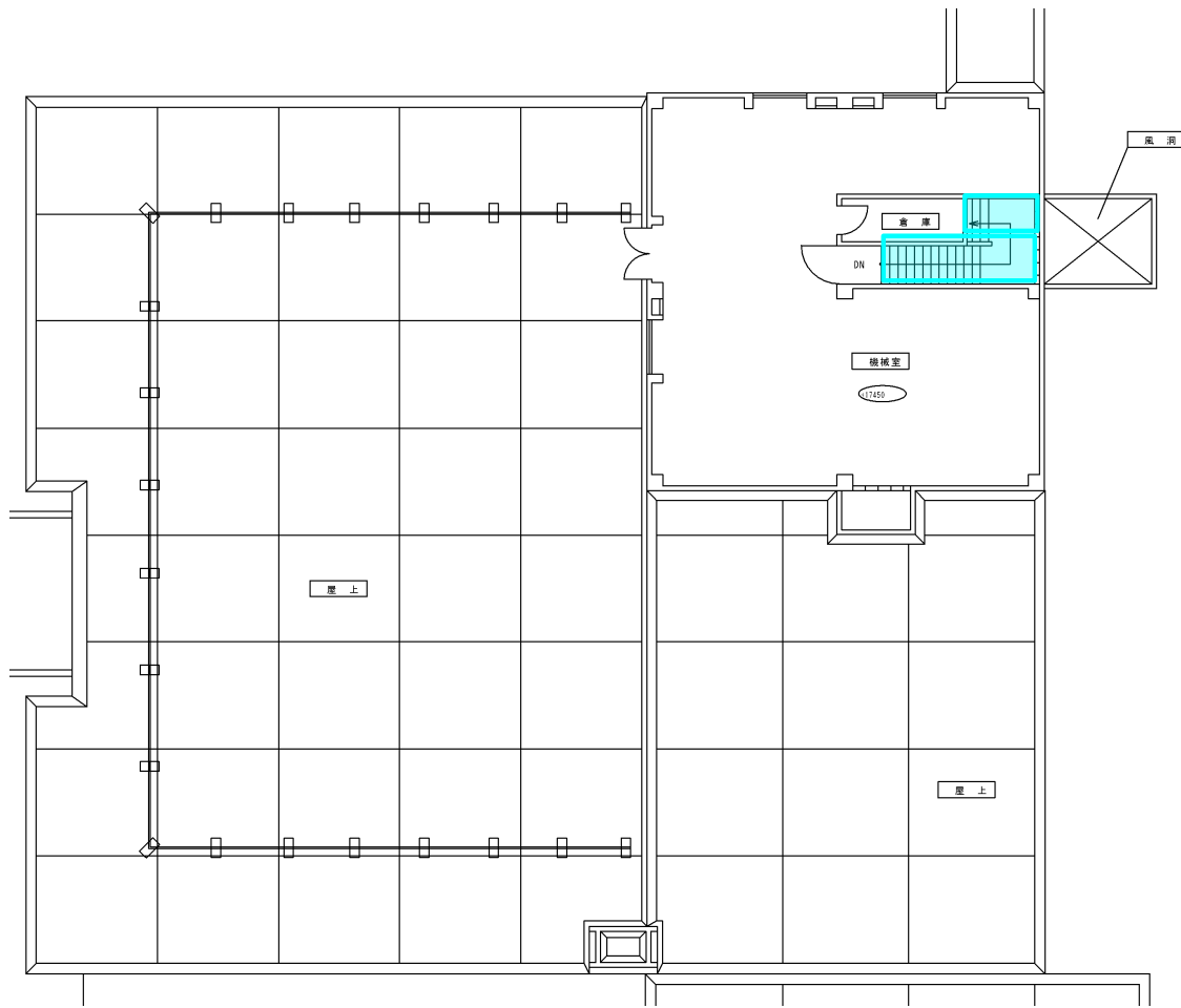
本館3階 S=1:200
