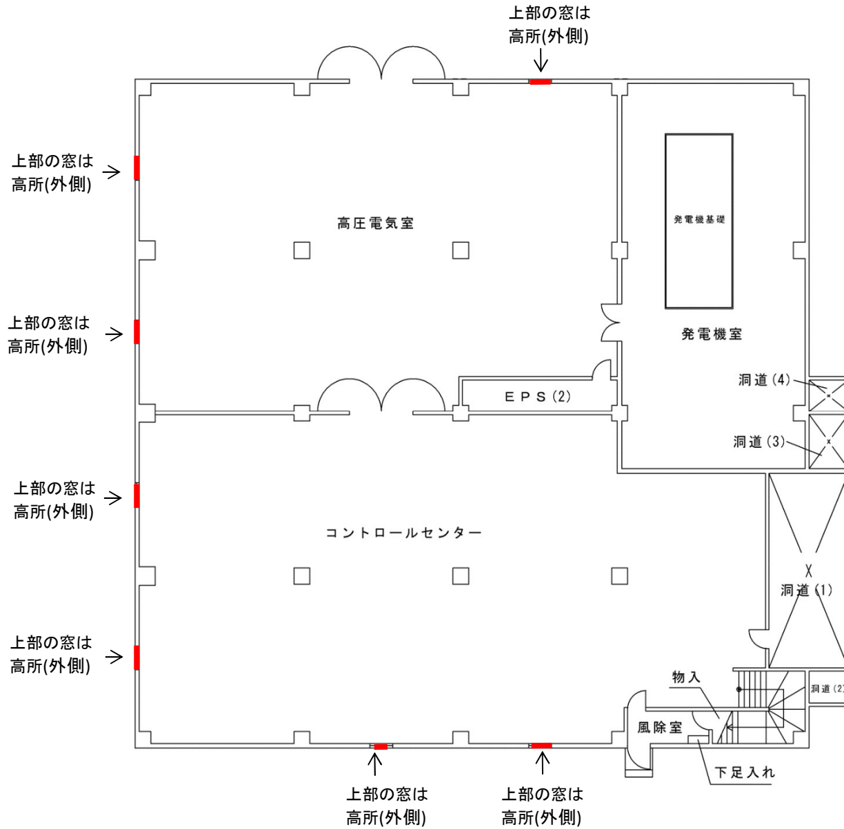
新館1階 S=1:200
