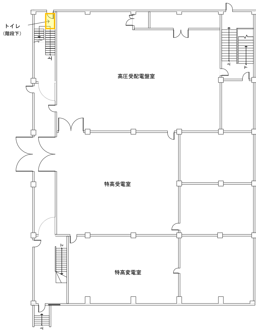
第2処理施設1階 S=1:200
