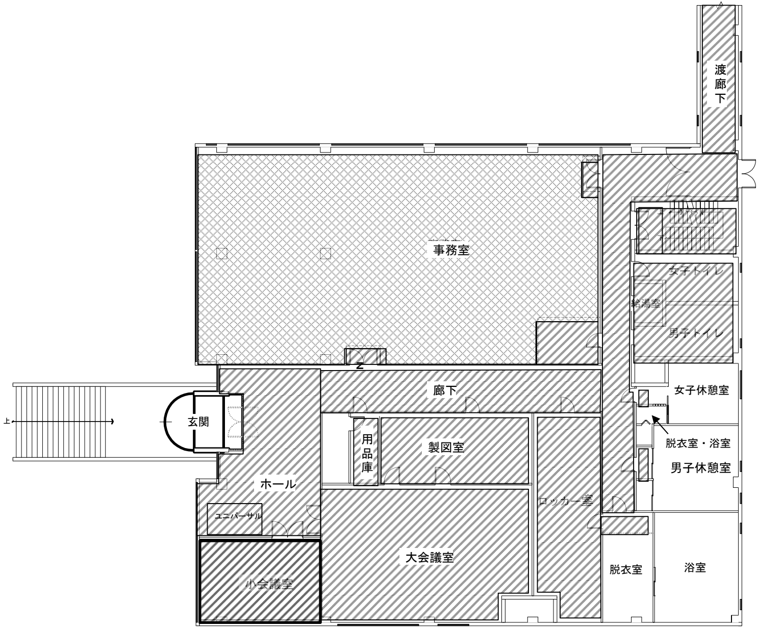
本館2階 S=1:200
