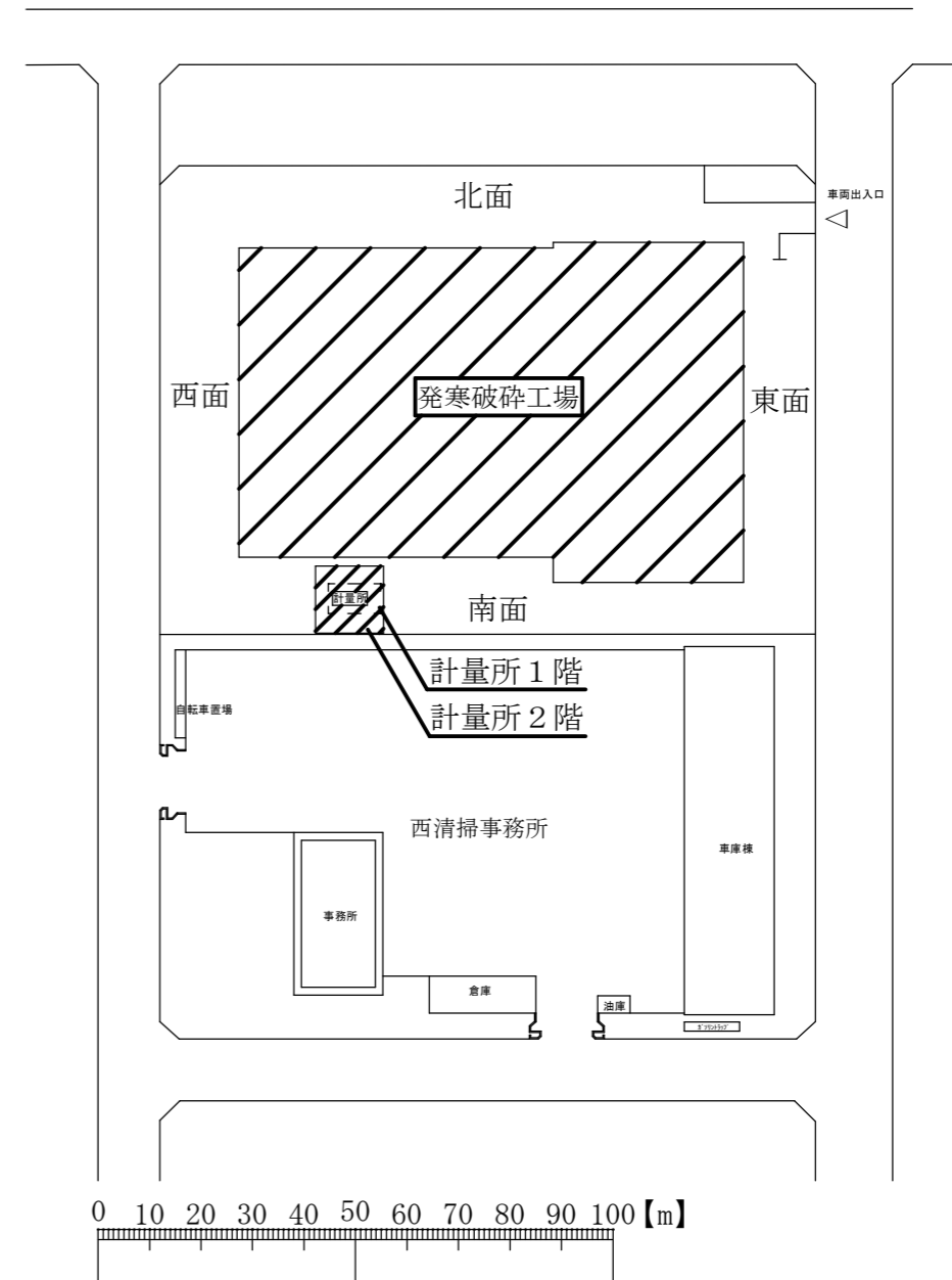
配置図 1/1,500
