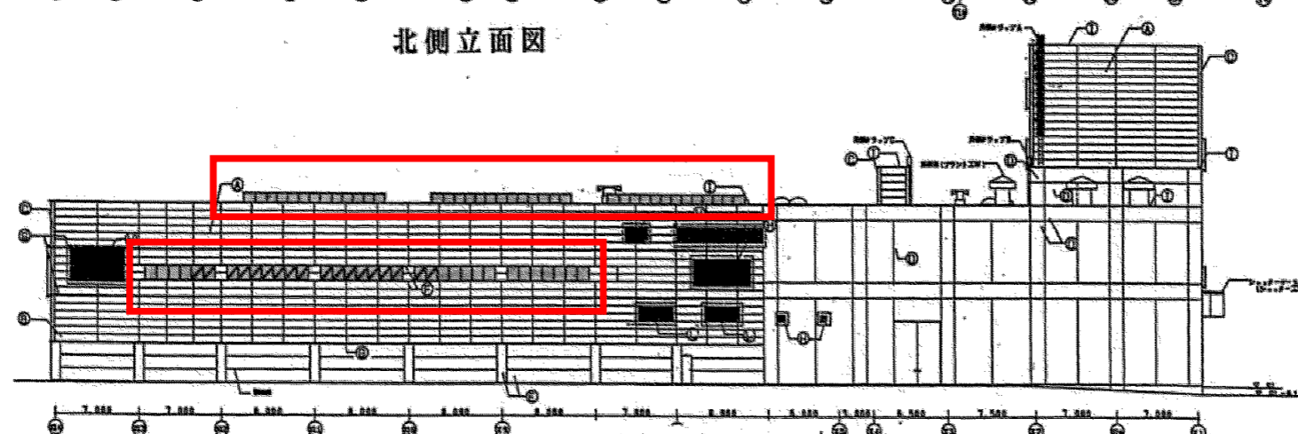
東側立面図
