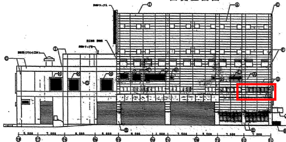
北側立面図
