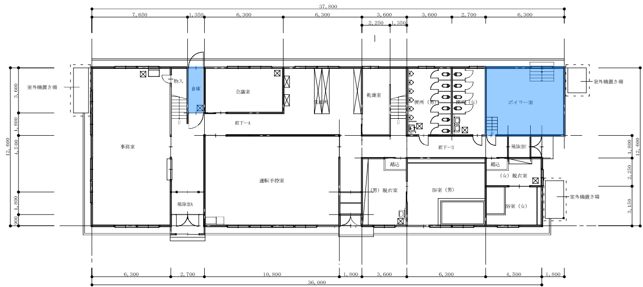
1 階平面図
