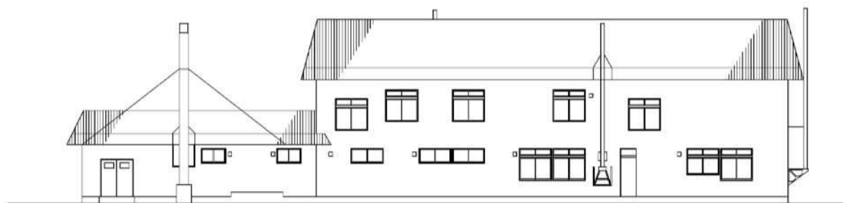
北側立面図
