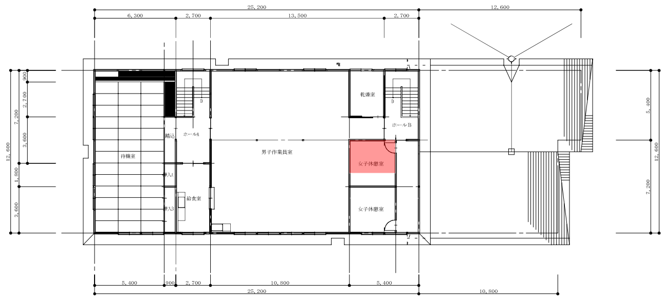
2 階平面図
