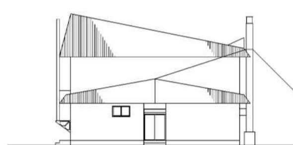
東側立面図
