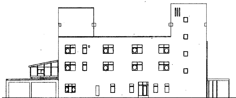
北立面图
