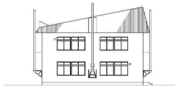
西側立面図
