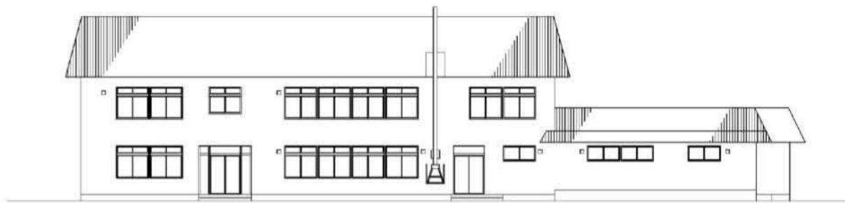
南側立面図
