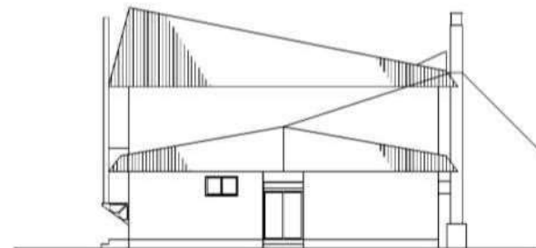
東側立面図
