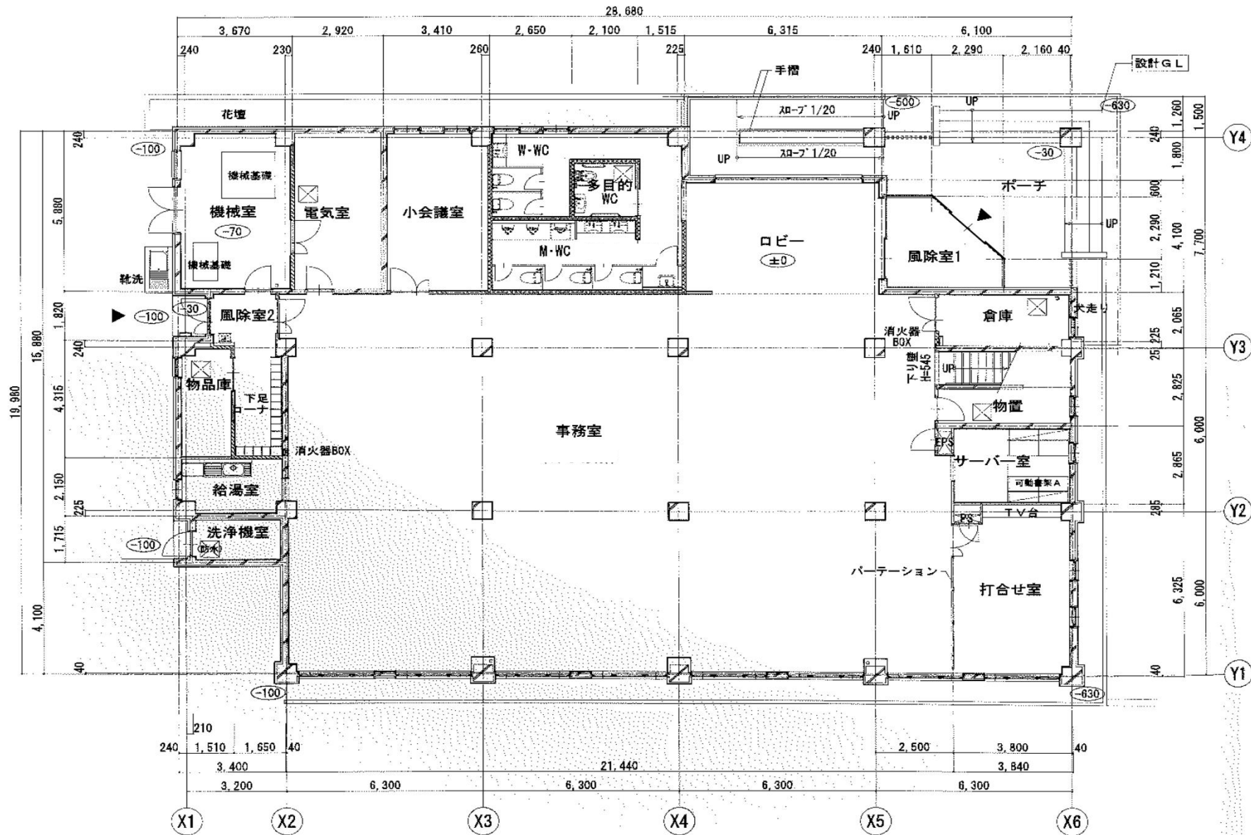
【豊平区土木センター平面図】
