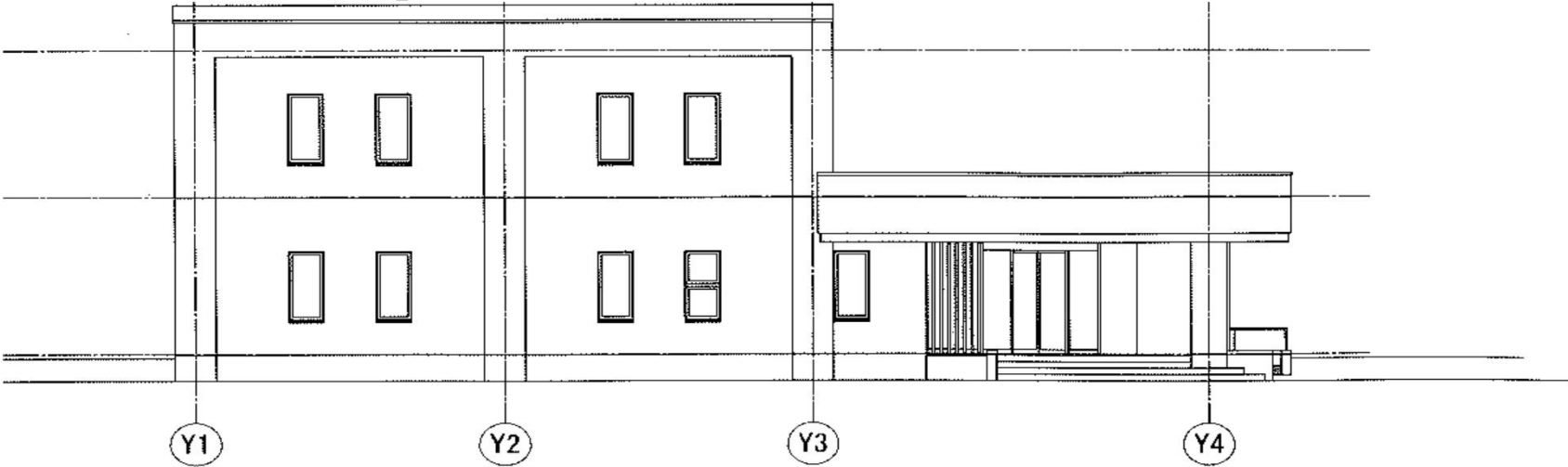
東側立面図
