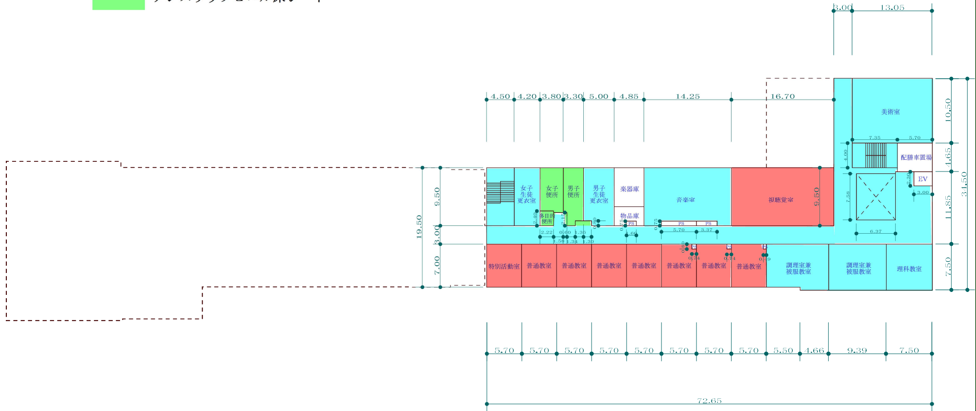
3階平面図
