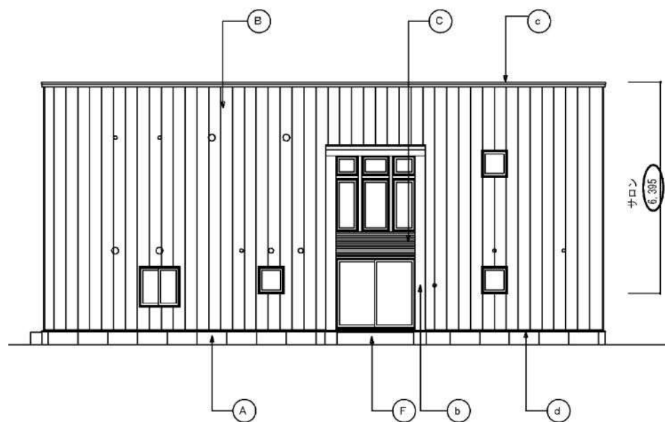
北面立面图
