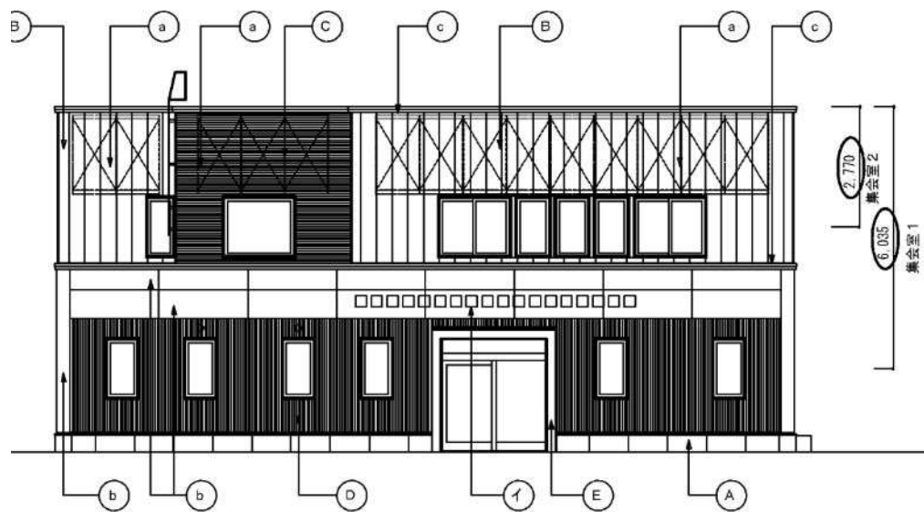
南面立面图
