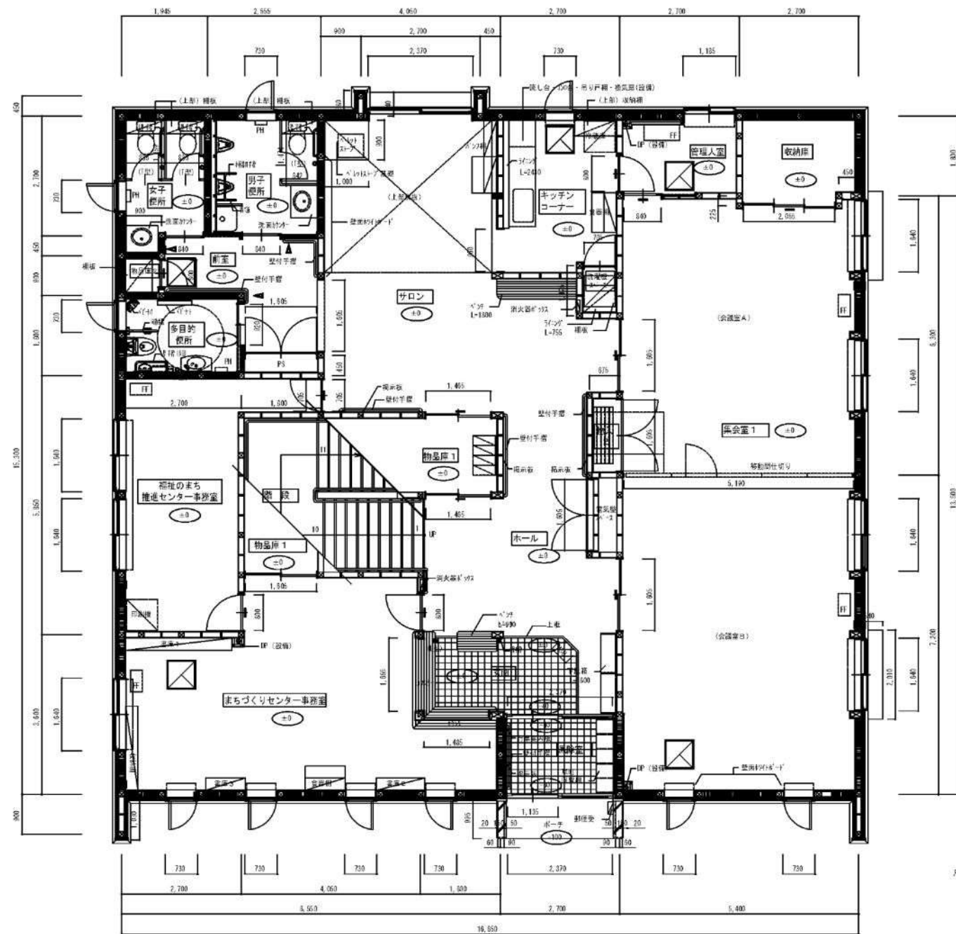
1 階平面詳細図
