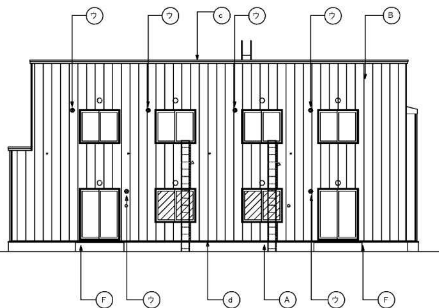
東面立面图
