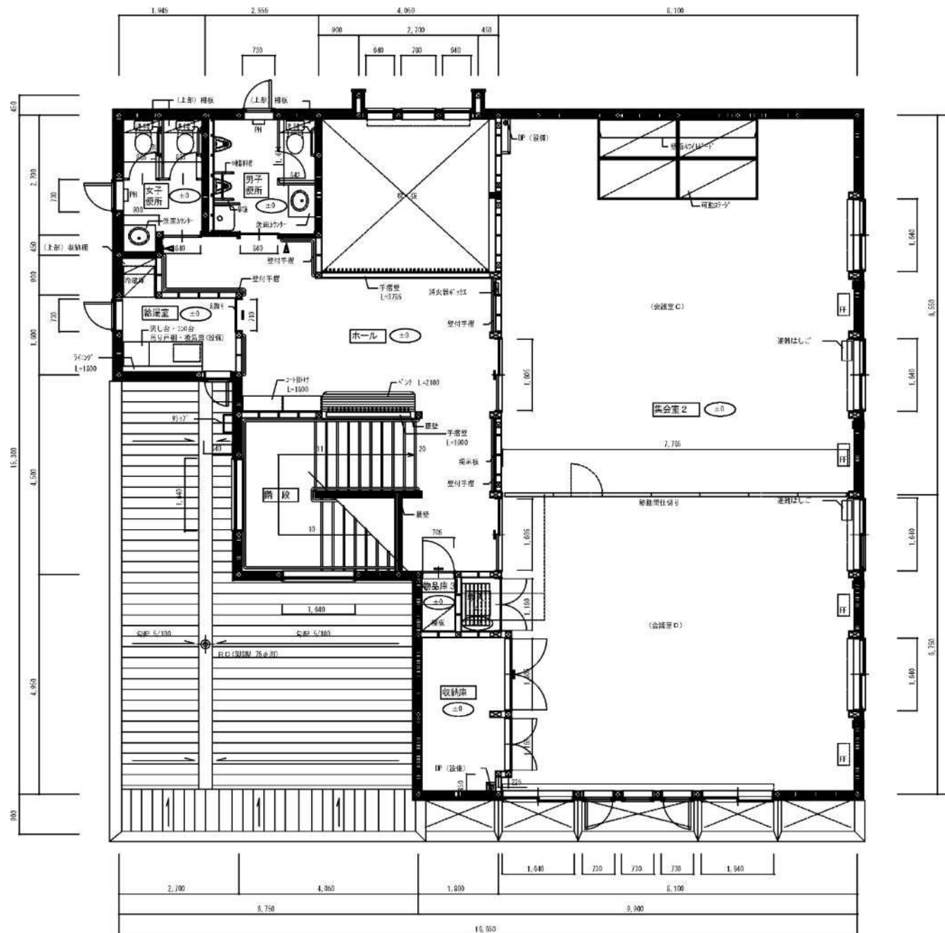
2階平面詳細図
