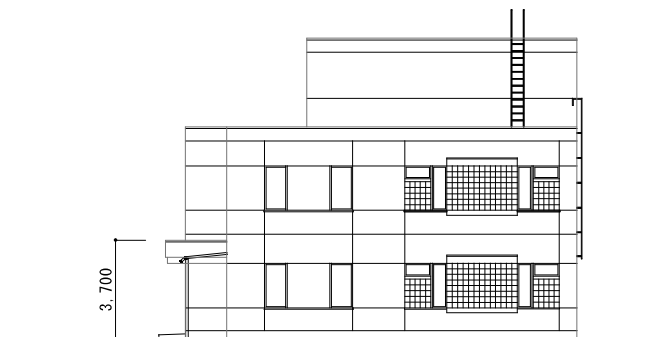
右側面図 S : 1/200
