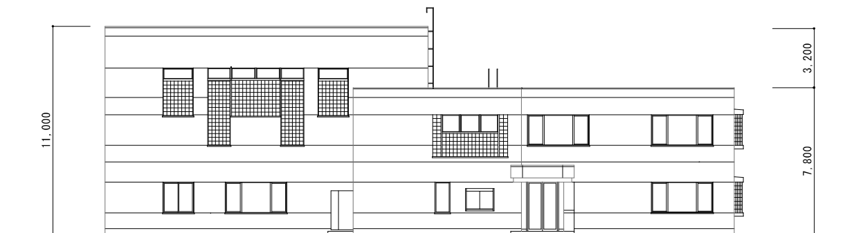
正面図 S : 1/200
