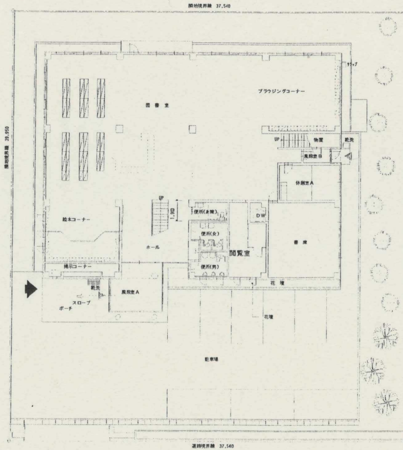
配置図・1階平面図
