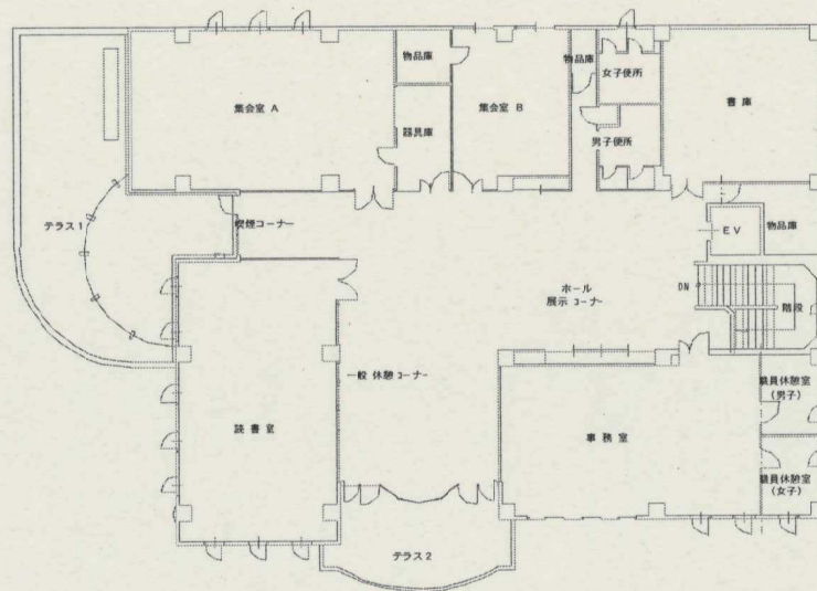
2階平面図
