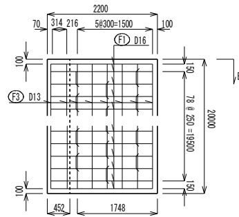
底板下面 D-D
