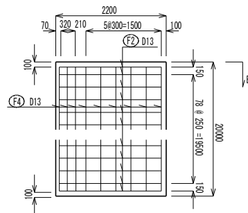
底板下面 D-D
