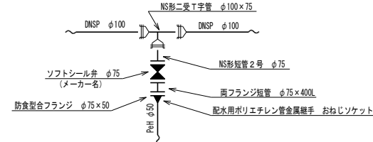
D部詳細図
