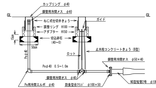
排水装置設置標準図
