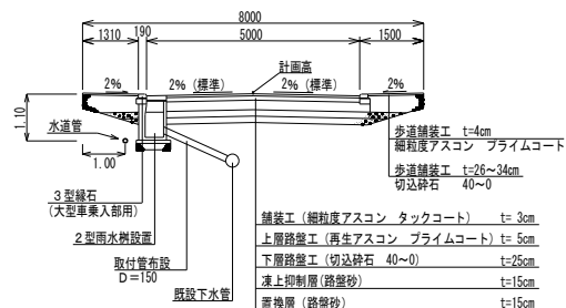
土工定規図 s=1:000
