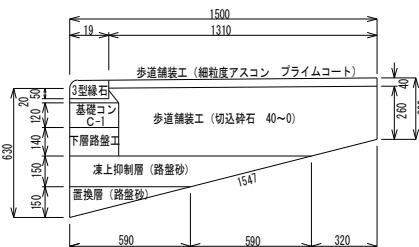
歩道部詳細図 s=1:000
