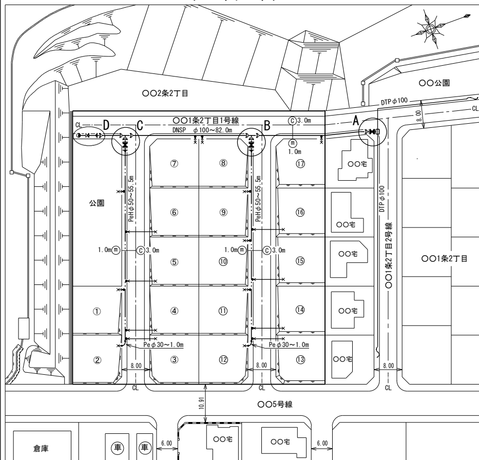
平面図 1:500
