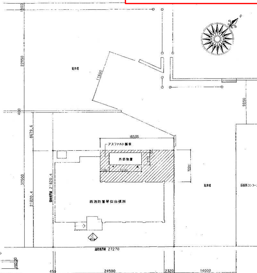
配置図 1:200
