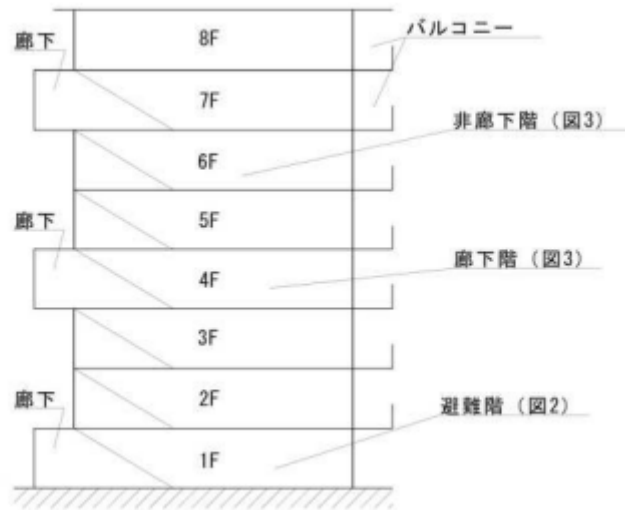
図4 断面例
