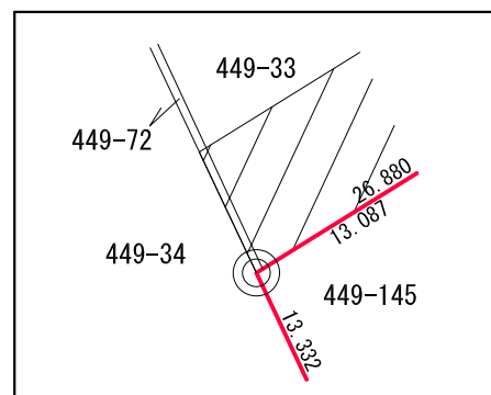
拡大図 A S=1/200
