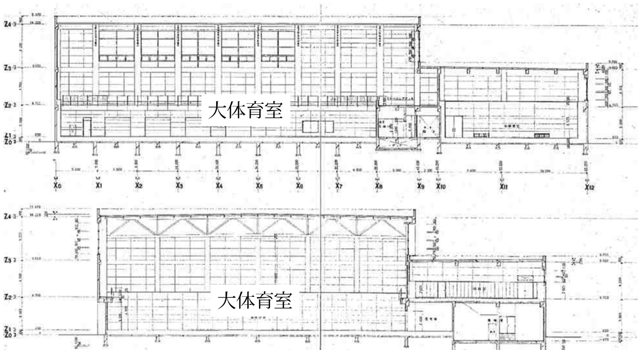
断面圖
