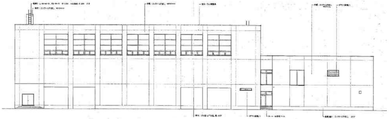
南側立面圖
