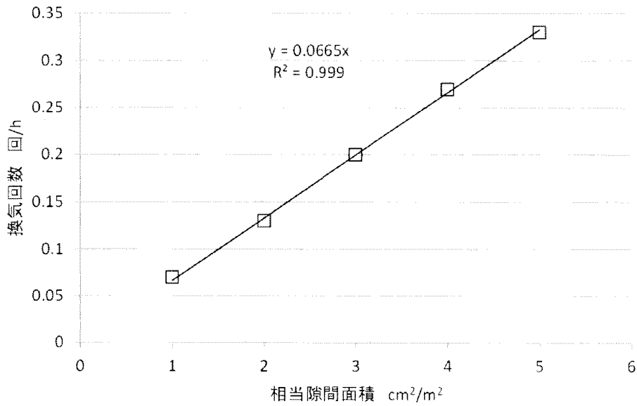
図1. 内外温度差20°C(外気平均0°C、室温平均20°C)とした場合の相当隙間面積と換気回数の関係
