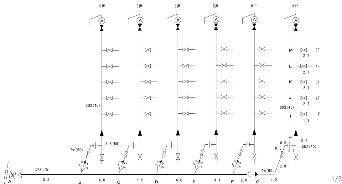
[5階直結給水(30戸)の例]
