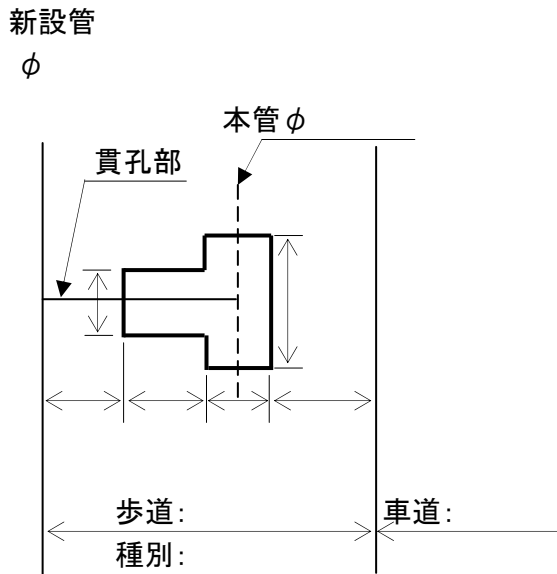
平面図
