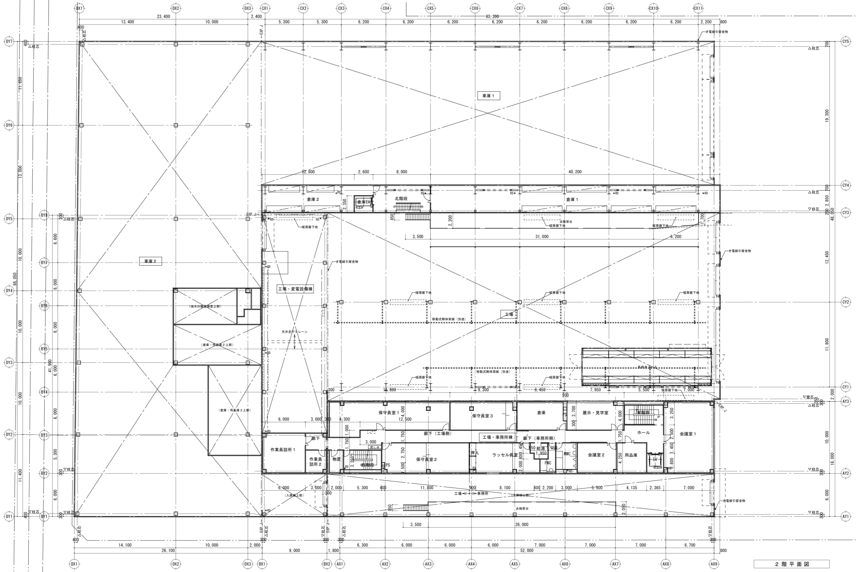
別紙4 新庁舎2階平面図
