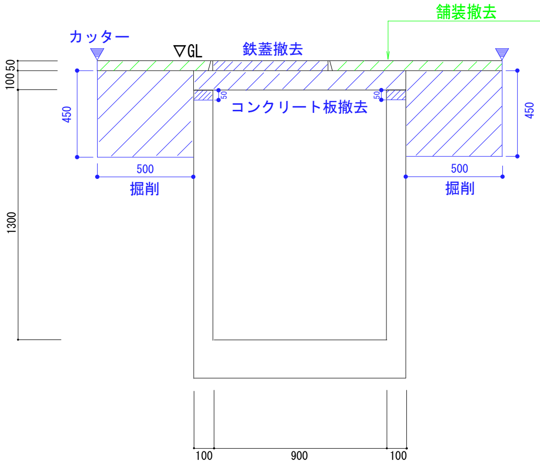
撤去図（正面・側面）
