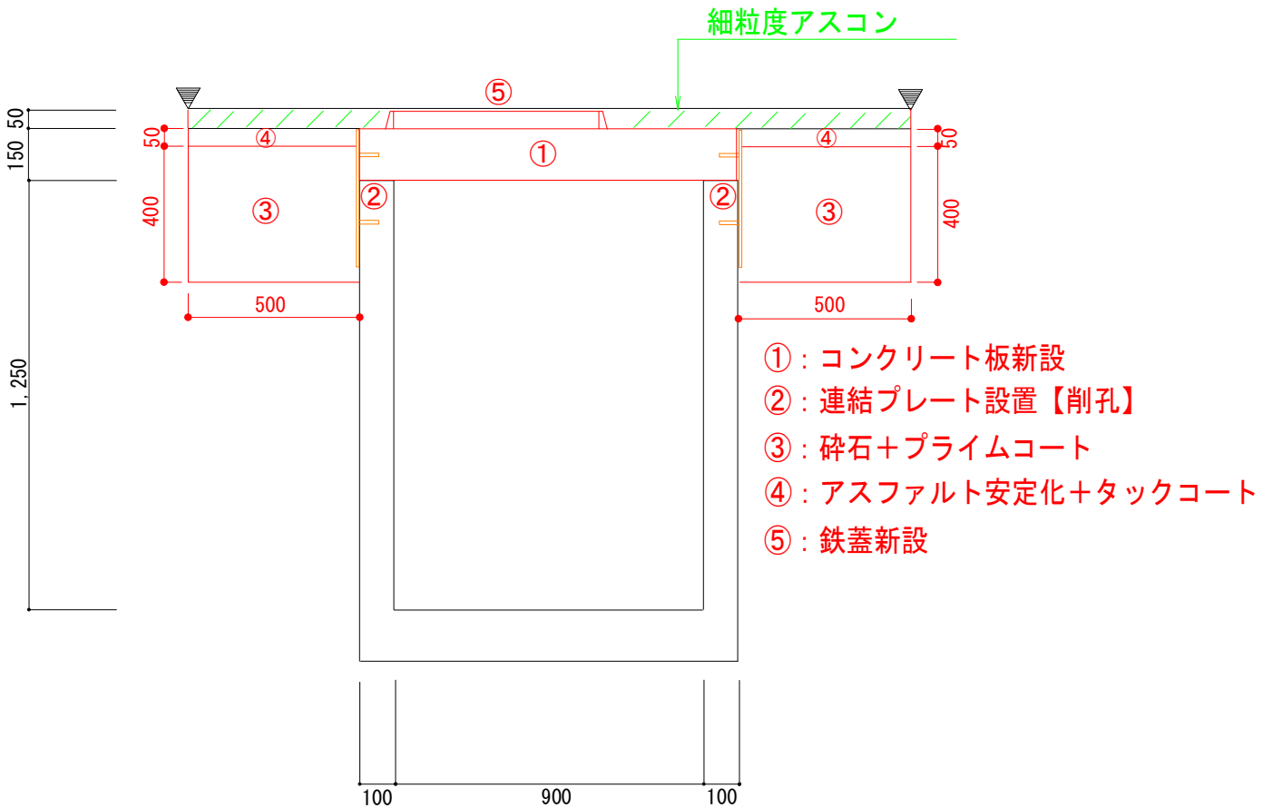
新設図（正面・側面）
