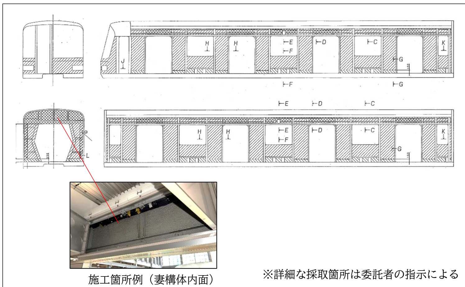
アンダーシール塗布箇所（構体内面）
