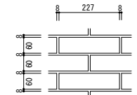
タイル標準目地詳細 ※貼替えタイルは既存類似色とする事。
