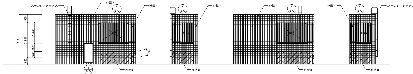
北立面図 1/100
