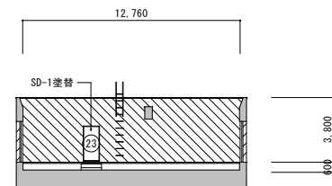
A 棟R00F2西側立面図
