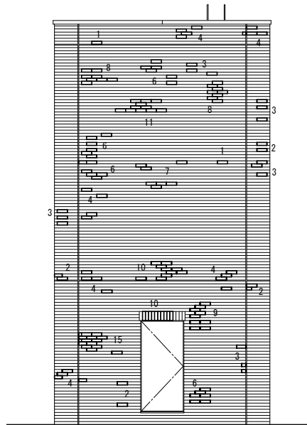
東側立面図 1/60 (タイル劣化図)
