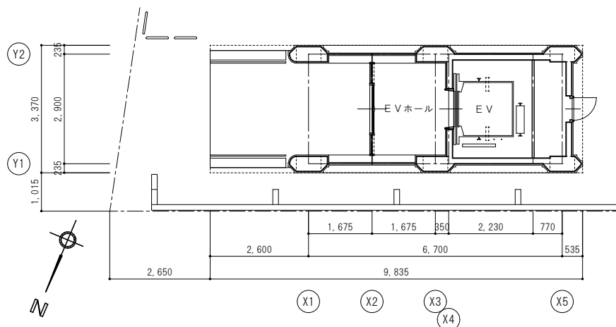
平面図 S : 1/100
