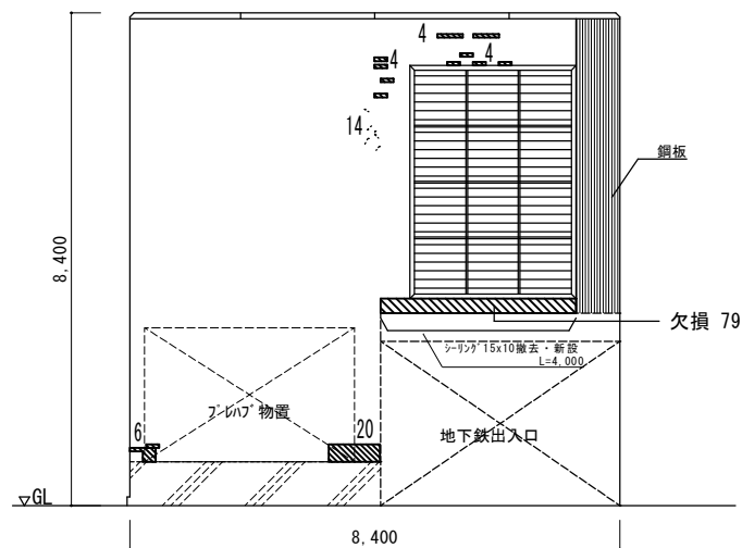
南 立面図
