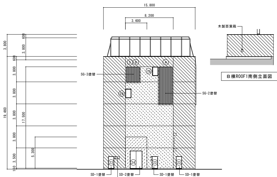
B棟南側立面図
