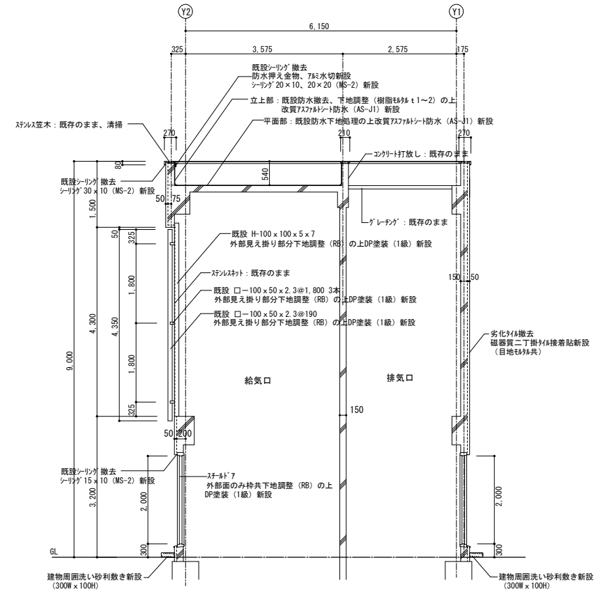
断面図 1/60
