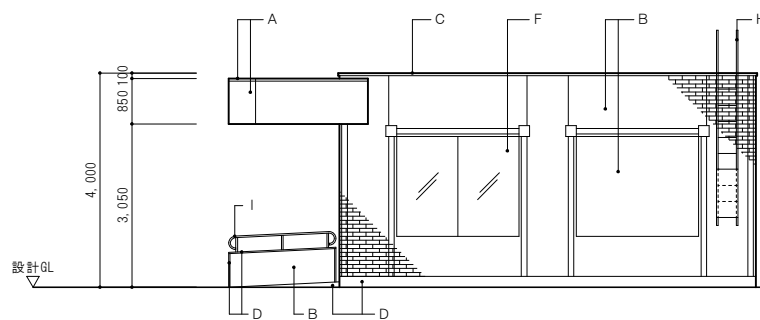
北面立面図 S : 1/100
