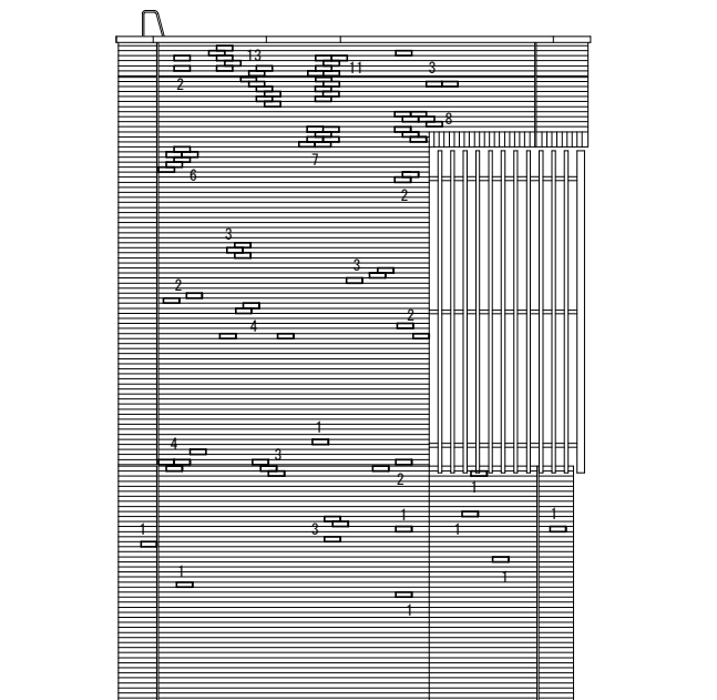
北側立面図 1/60 (タイル劣化図)
