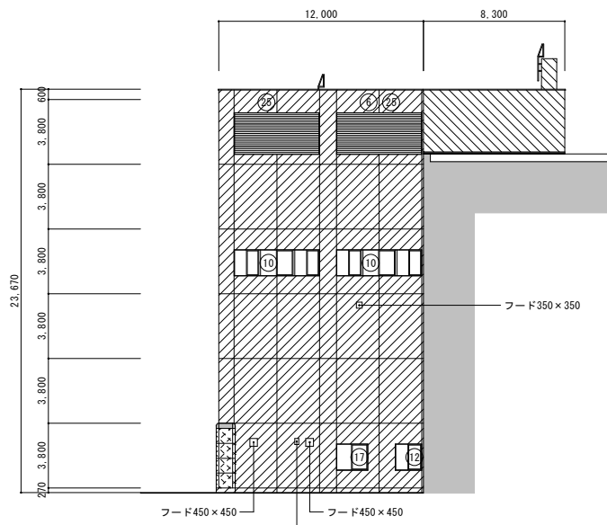
A 棟南側立面図
