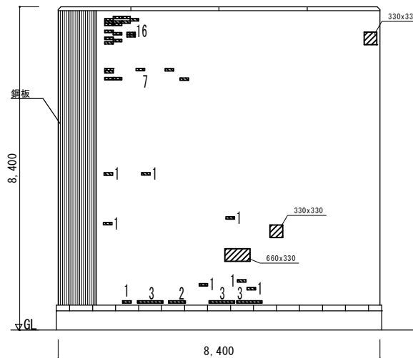
北 立面図
