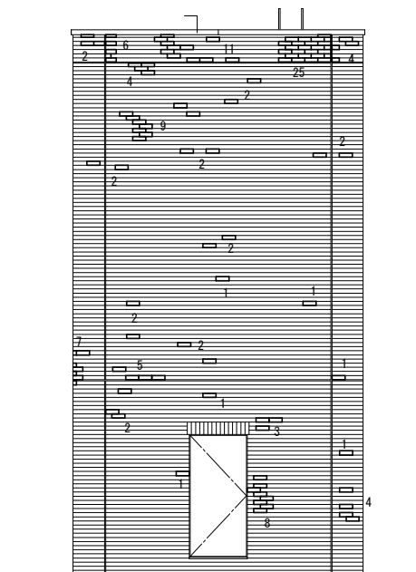
東側立面図 1/60 (タイル劣化図)
