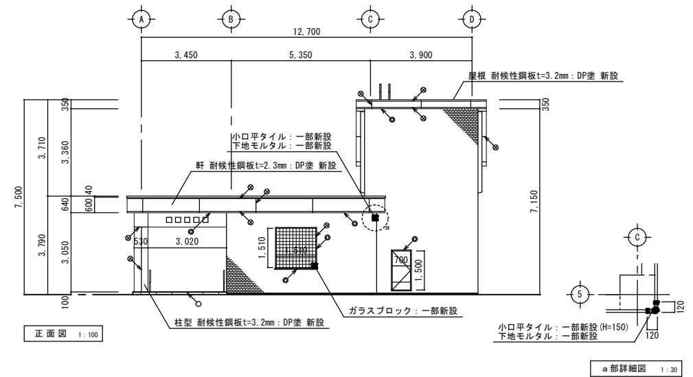
改修後 1番出入口 立面図-1
