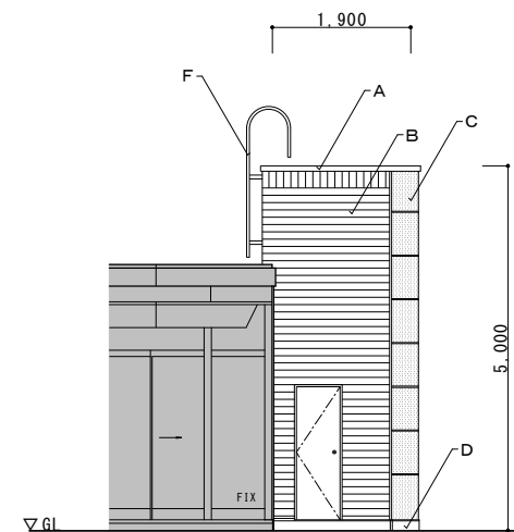
東側立面図 S.1:50
