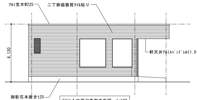
EV出入口現況西側立面図 1/100
