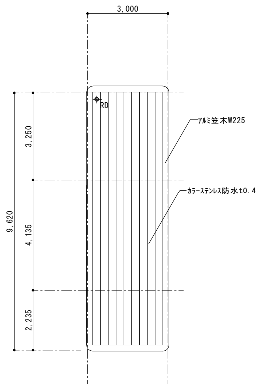
EV出入口現況屋上平面図 1/100
