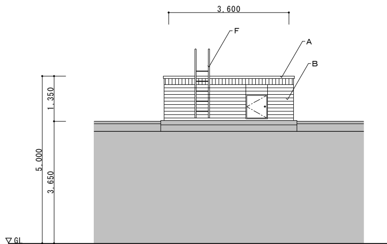
南側立面図 S.1:50
