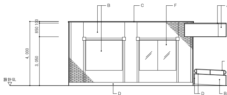
南面立面図 S : 1/100
