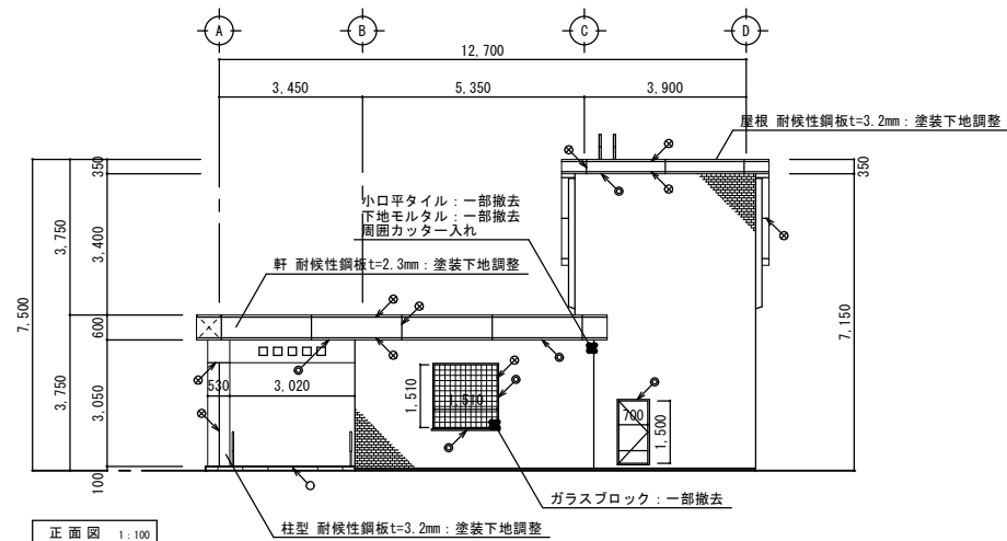
改修前 1番出入口 立面図-1
