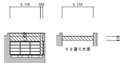
A 棟R00F2北側立面図
