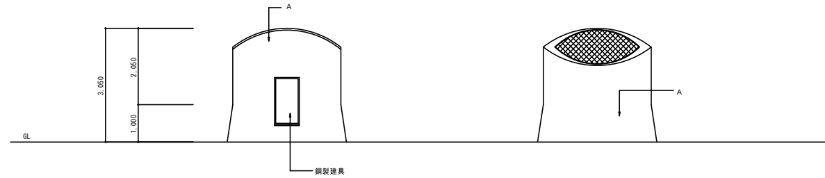
立面図-1 1/50
