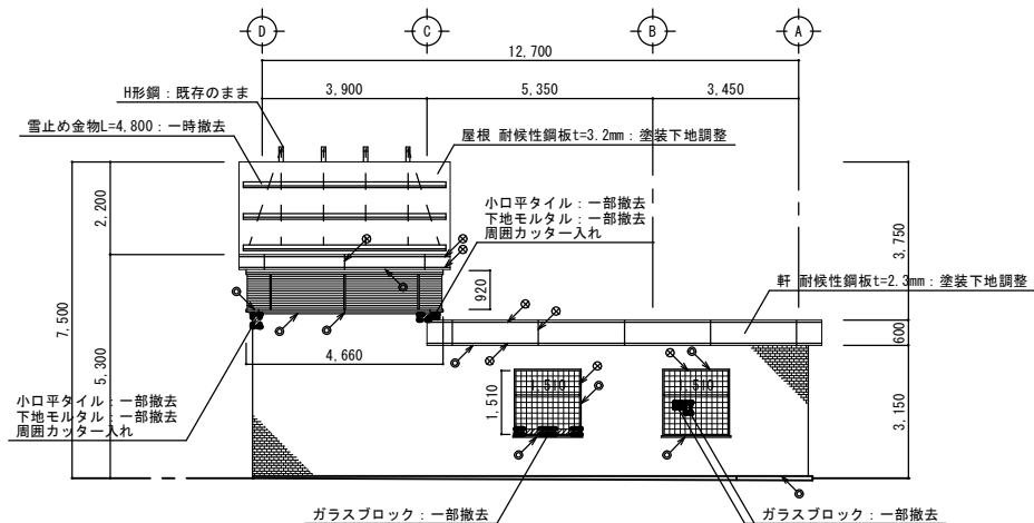
背面図 1:100
