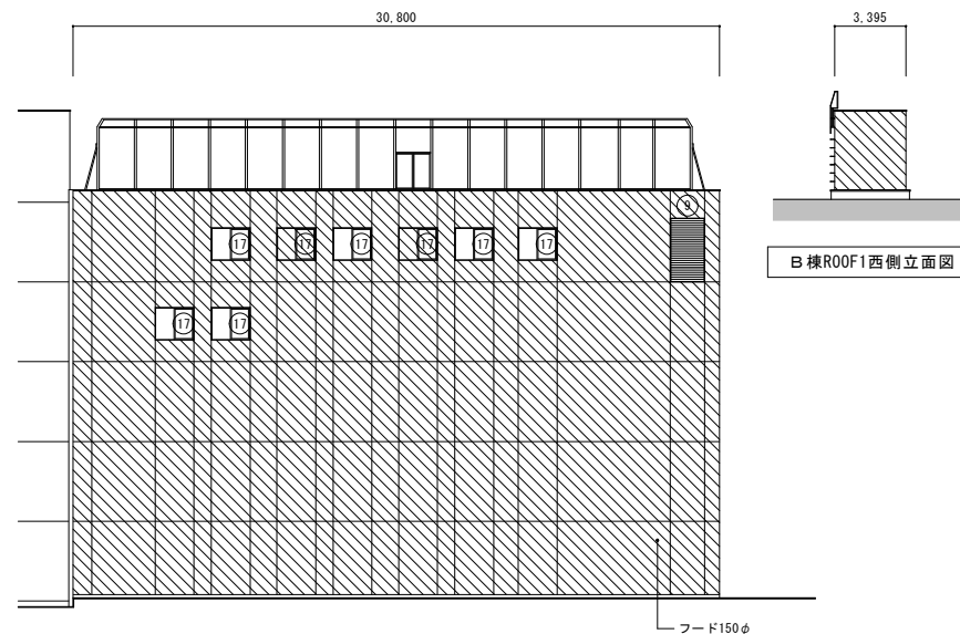
B棟西側立面図
