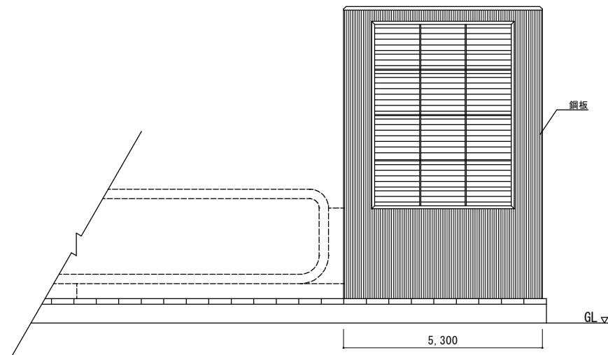
東 立面図
