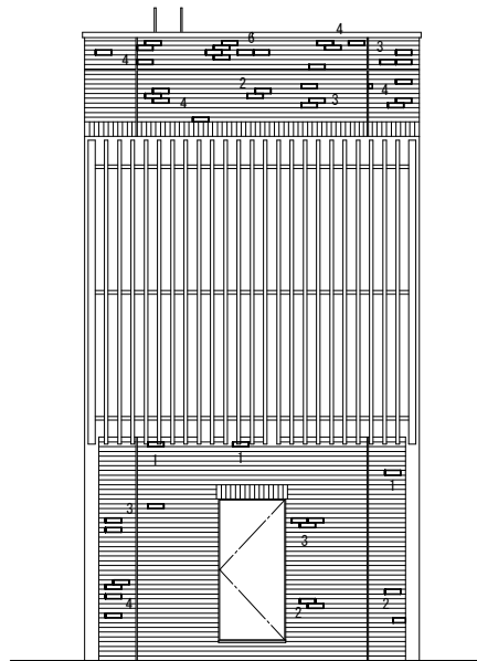
西側立面図 1/60 (タイル劣化図)
