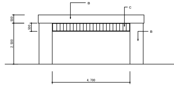
南 立面図 1/50
