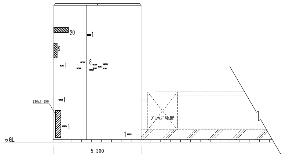
西 立面図
