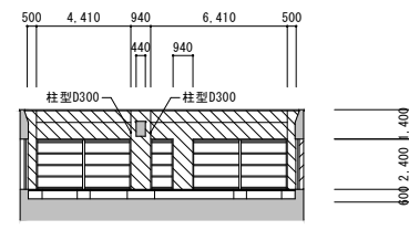
A 棟R00F2東側立面図
