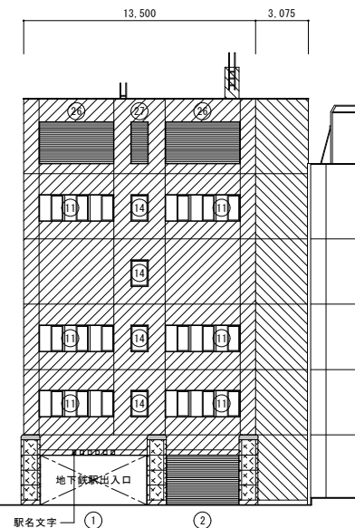
A 棟西側立面図
