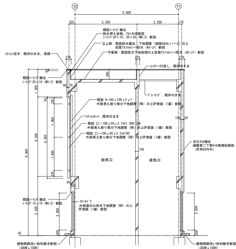
断面図 1/60
