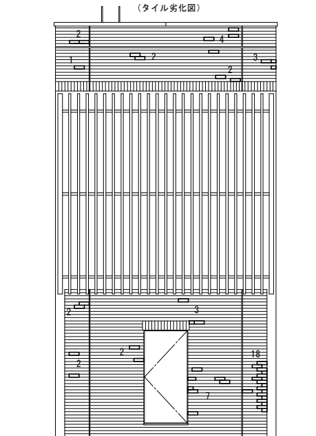
西側立面図 1/60 (タイル劣化図)
