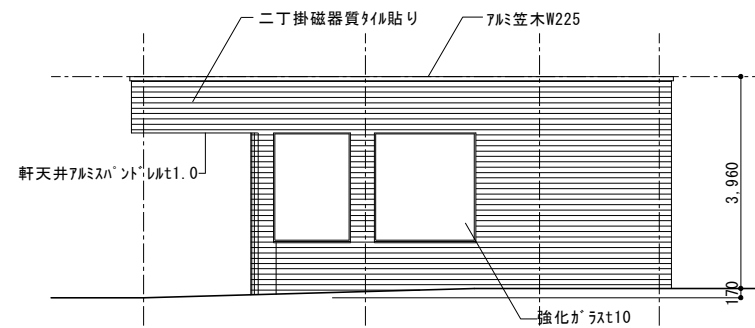
EV出入口現況東側立面図 1/100
