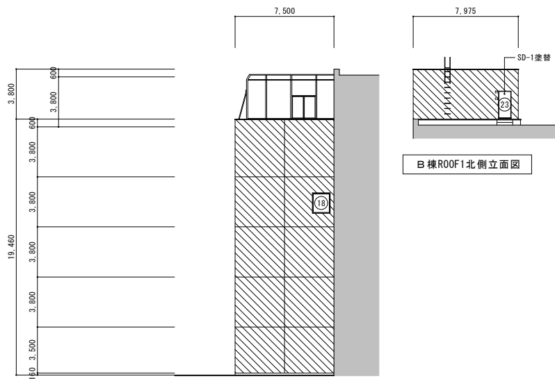
B棟北側立面図
