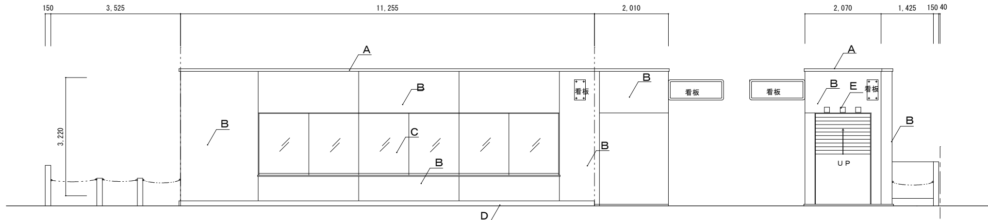
A 立面図
