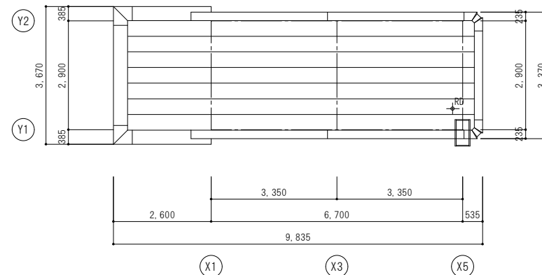
屋根伏図 S : 1/100
