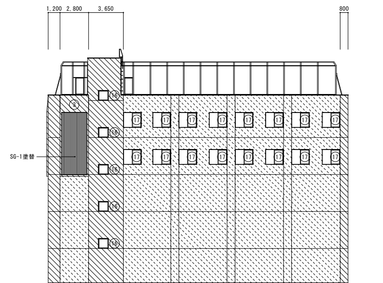
Ｂ棟東側立面図
