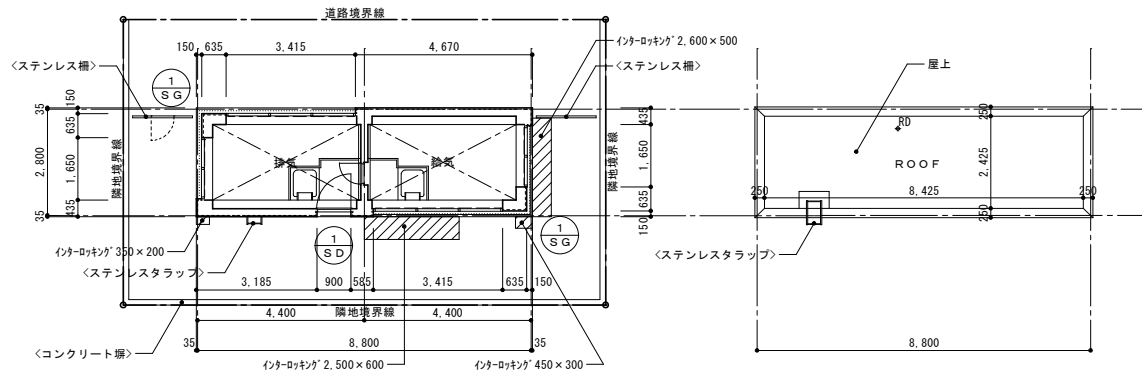
平面図 1/100
