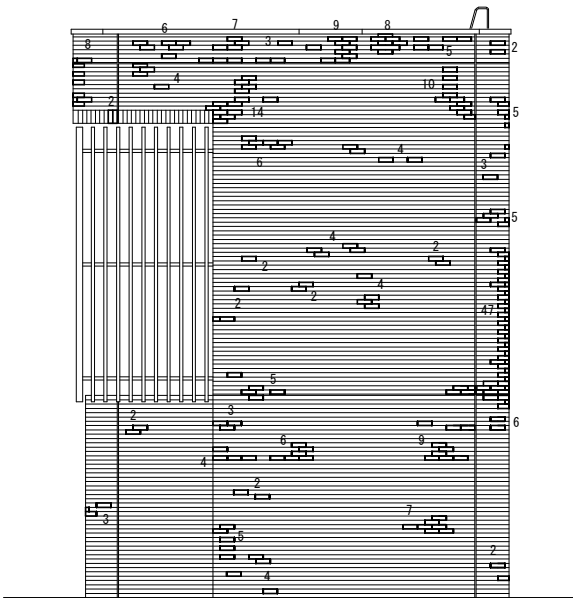
南側立面図 1/60 (タイル劣化図)
