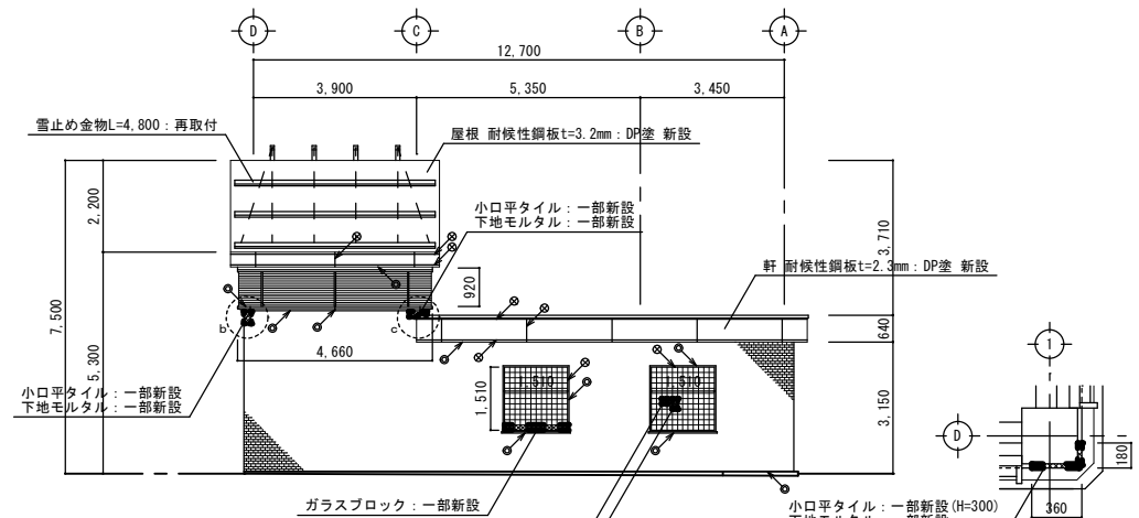
背面図 1:100
