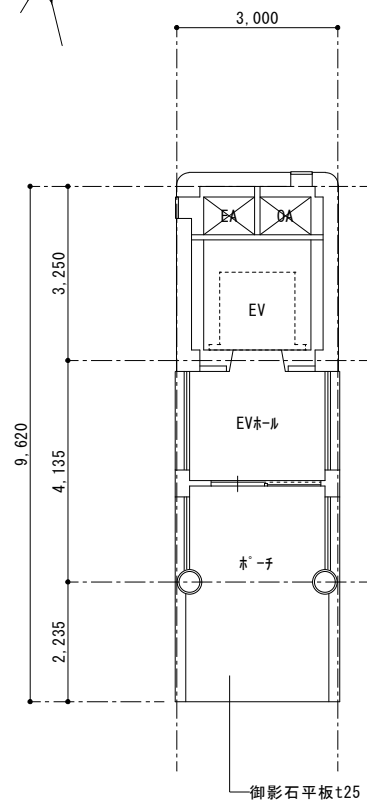
EV出入口現況平面図 1/100
