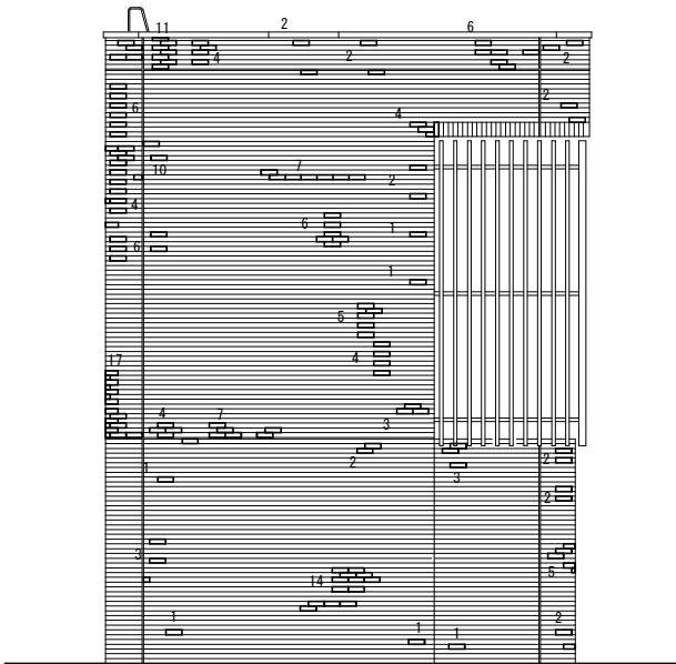
北側立面図 1/60 (タイル劣化図)
