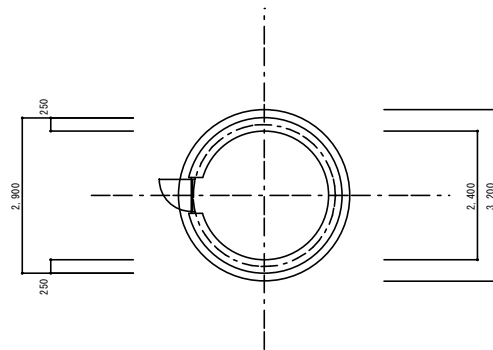
平面図 1/50
