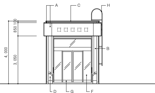
東面立面図 S : 1/100
