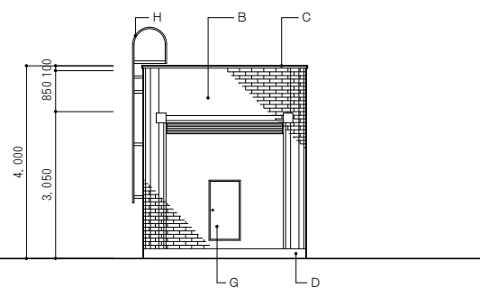
西面立面図 S : 1/100
