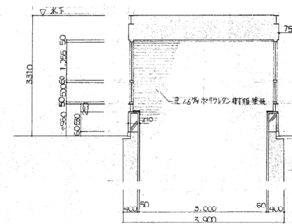
B-B 断面詳細図
