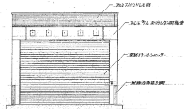
B 立面図
