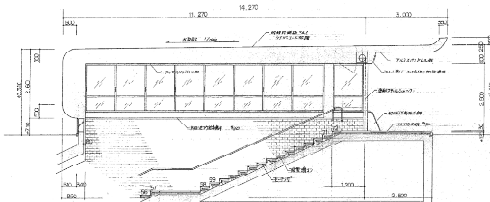
A-A 断面詳細図 1:100
