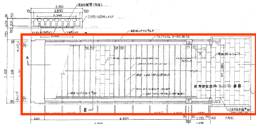
出入口平面図 1:100
