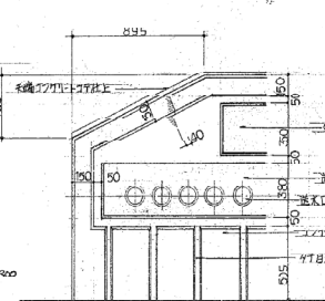
B-B 断面詳細図
