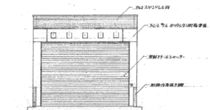
B 立面図
