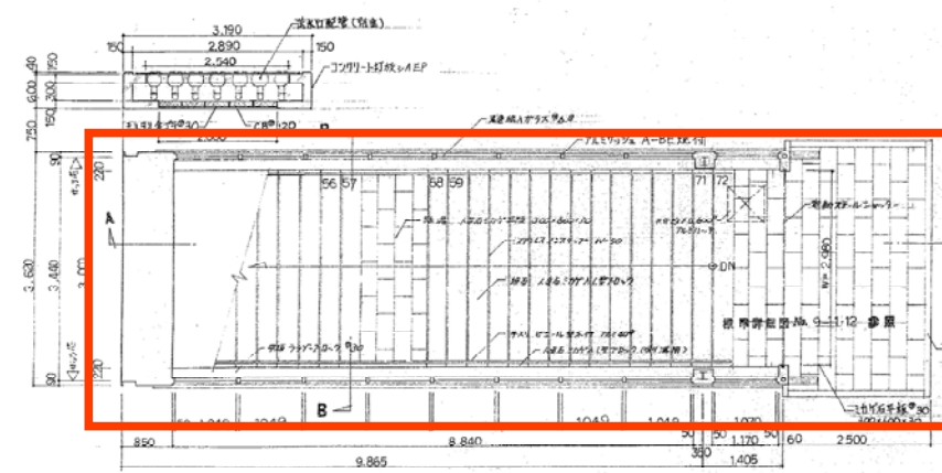
B 平面詳細図 1/100
