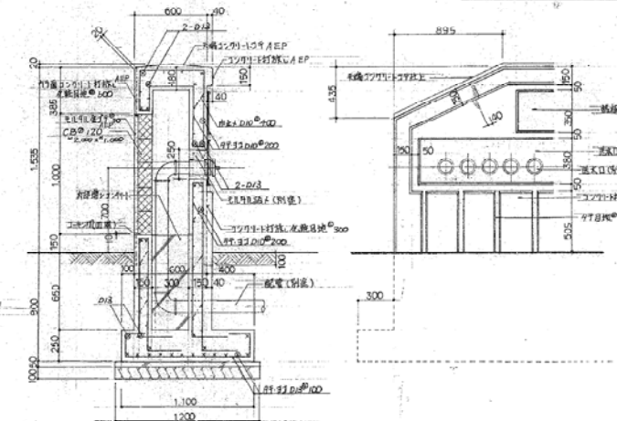
建物の水口詳細図 1/200
