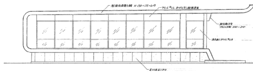
C 立面図 1/100
