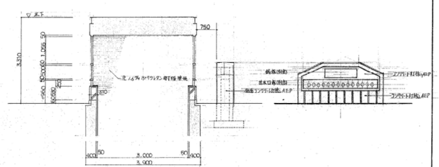
B-B 断面詳細図
