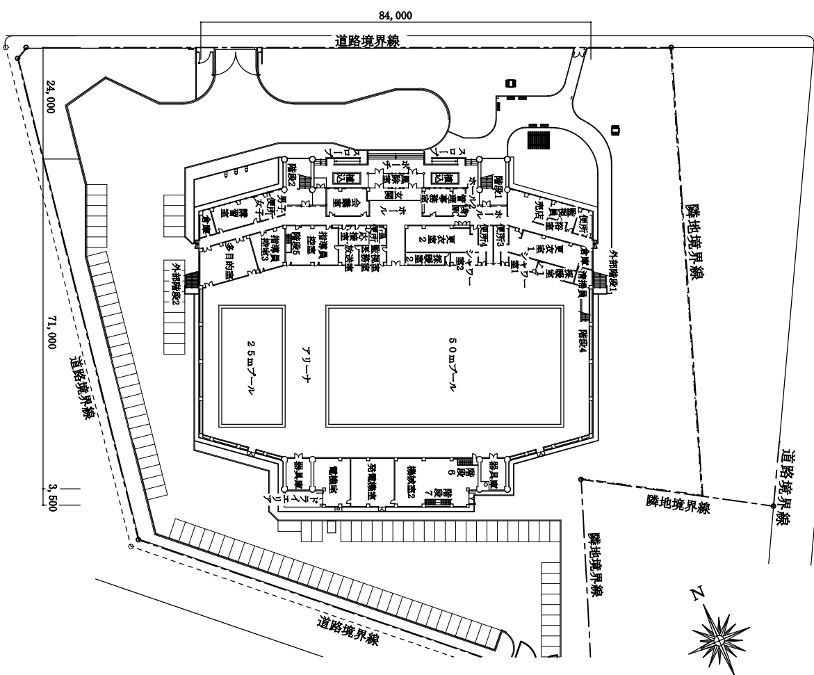
配置図
