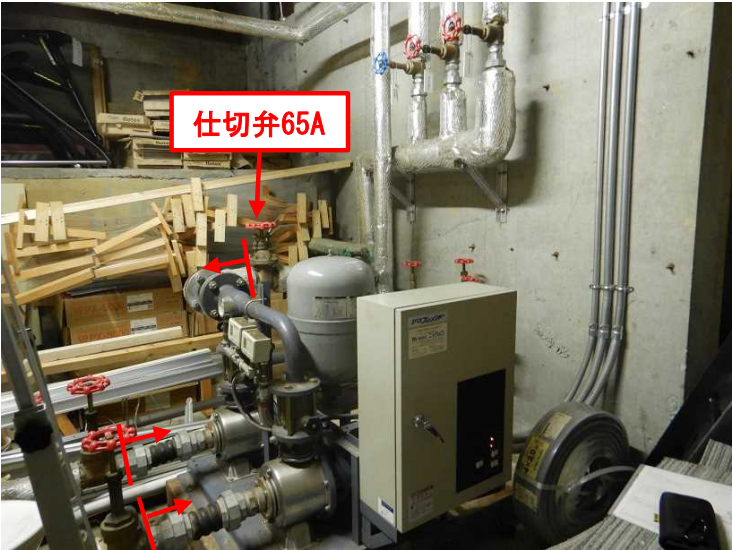
既設ポンプ（50UBPMD52.2）
