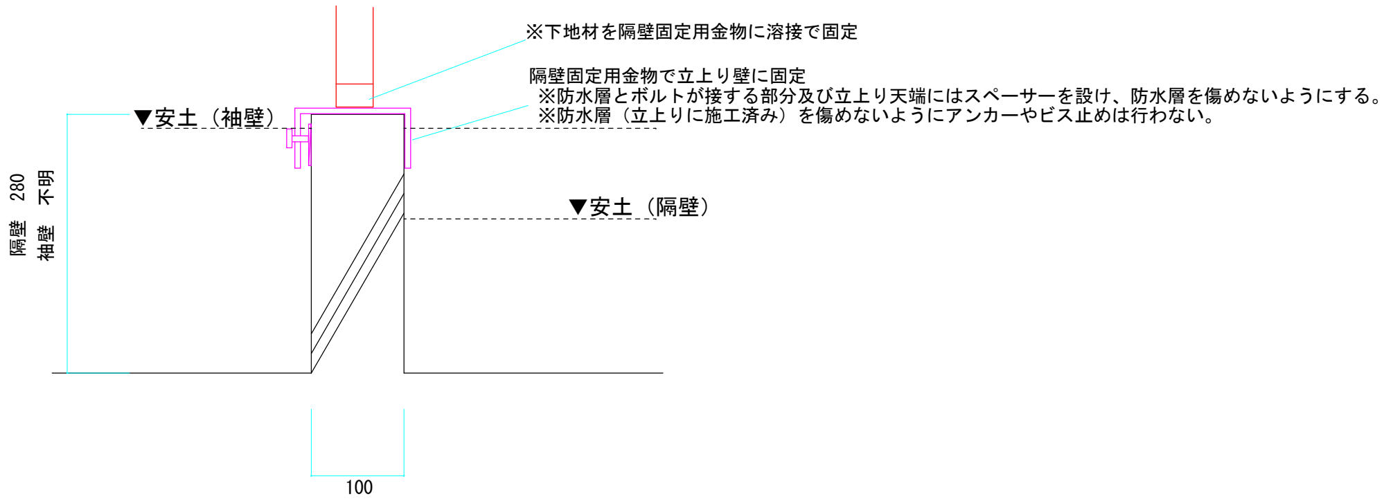
立上り詳細図
